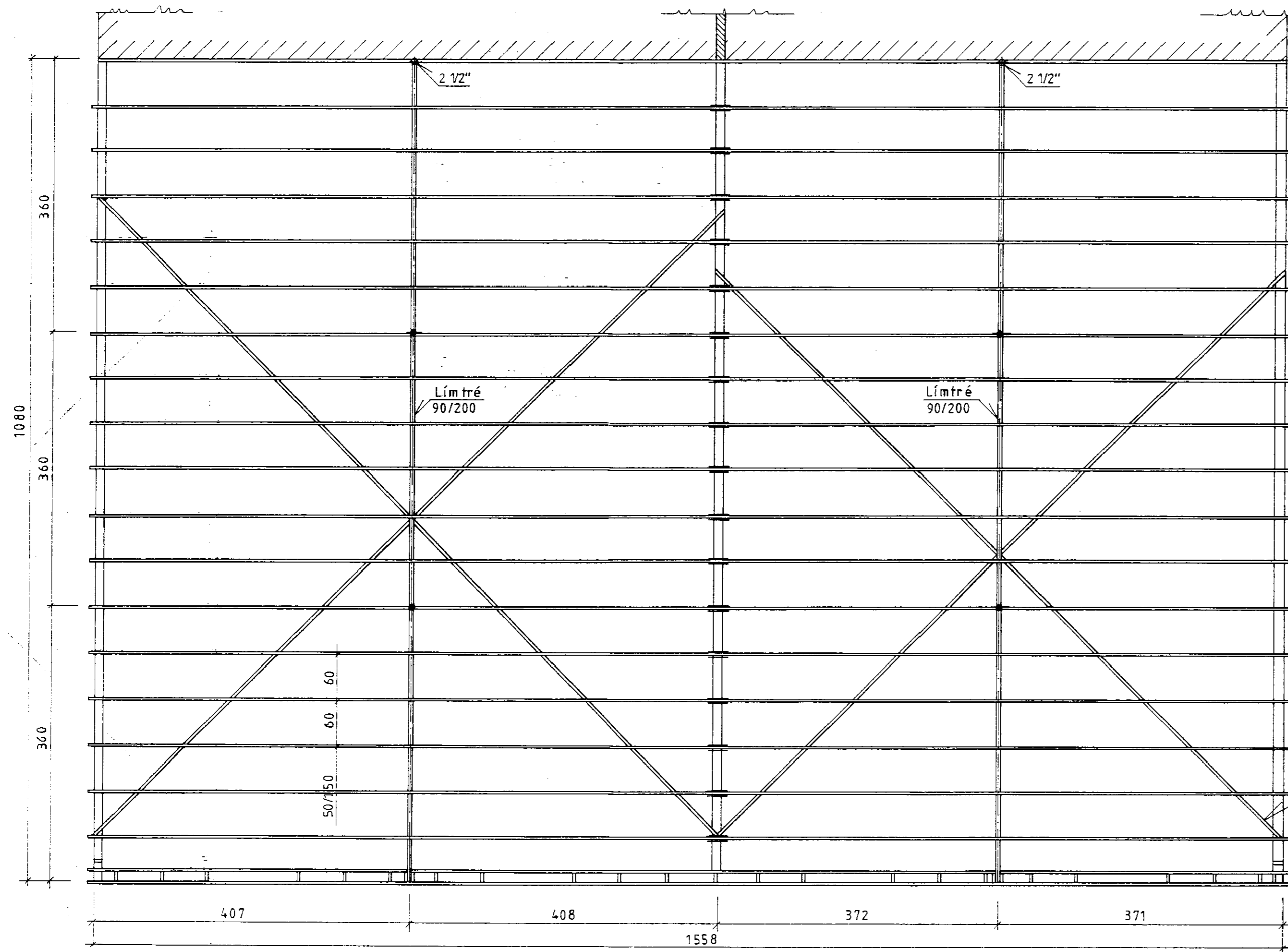
Pakgrunnmynd M = 1:50
