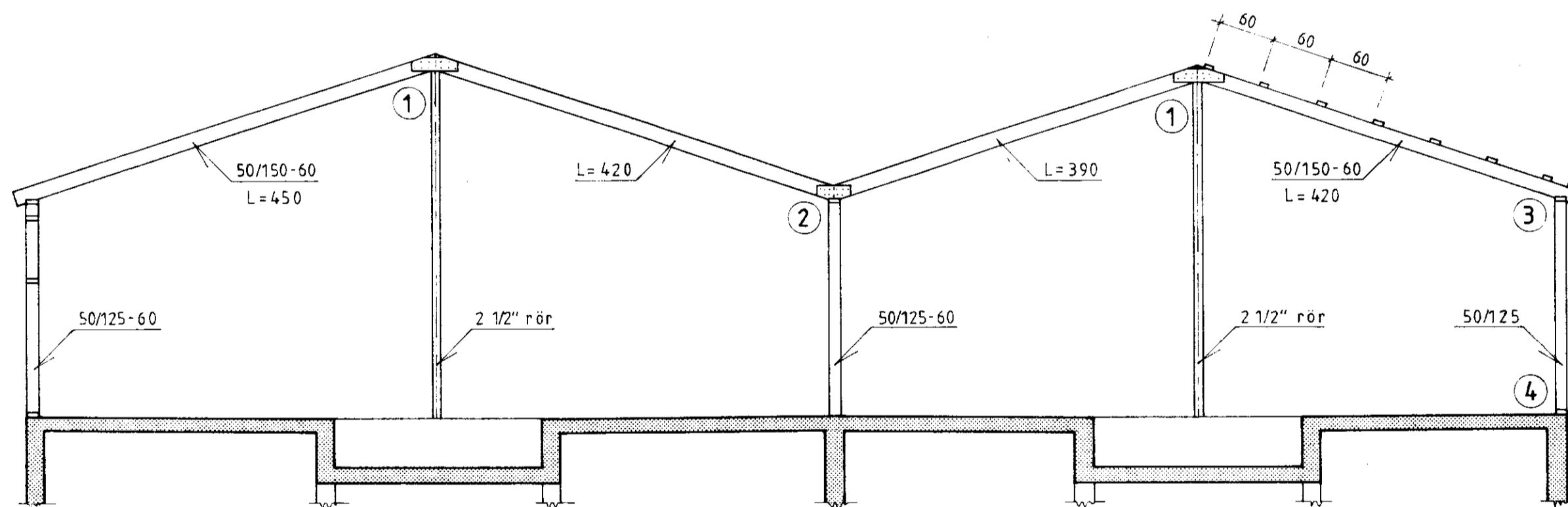
Þversnid M=1:50
