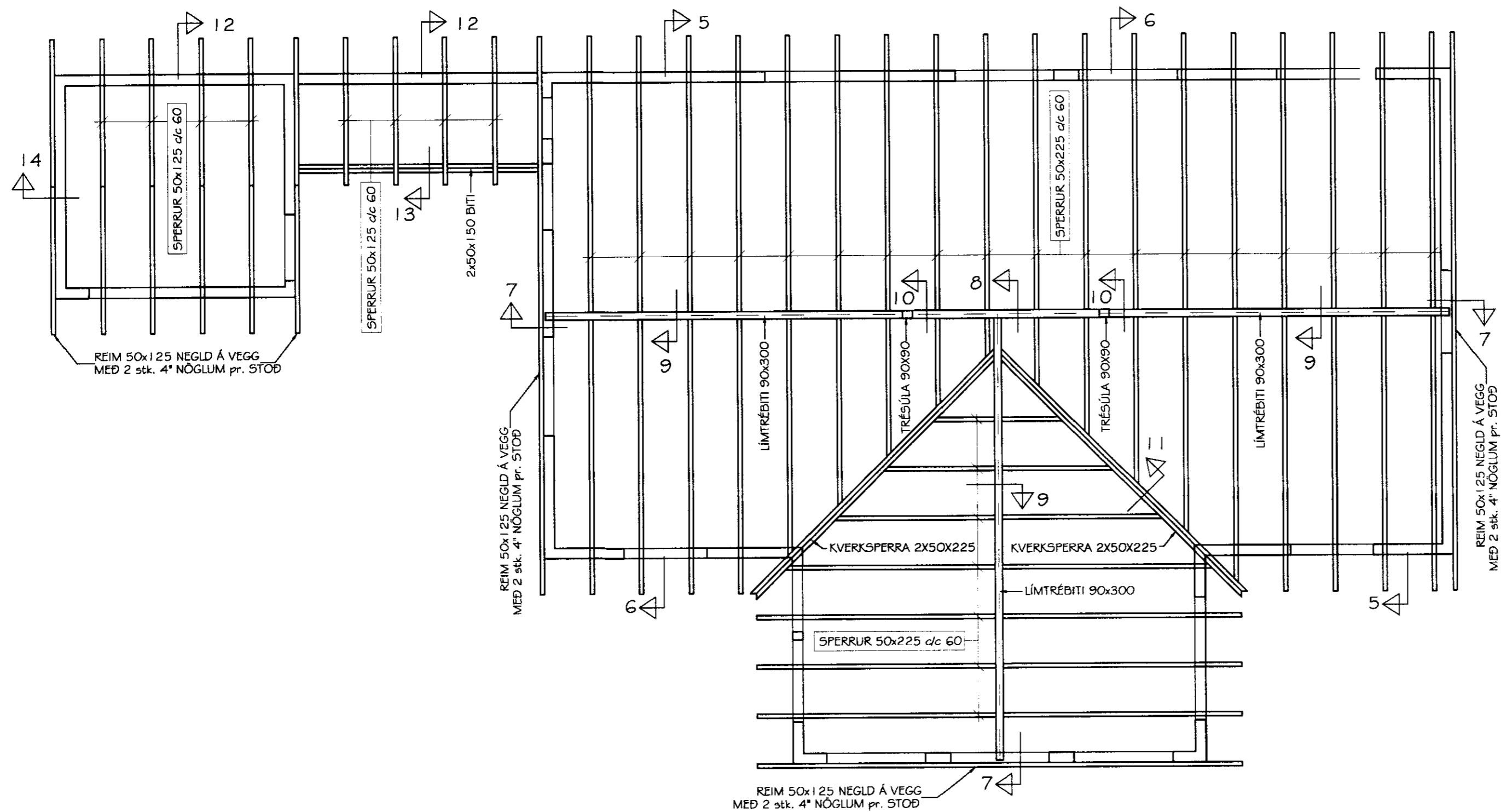
GRUNNMYND ÞAKVIÐA MKV. 1:50
