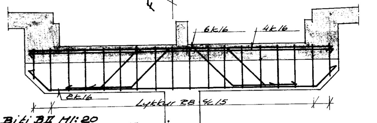
Bili B-B M1:20
