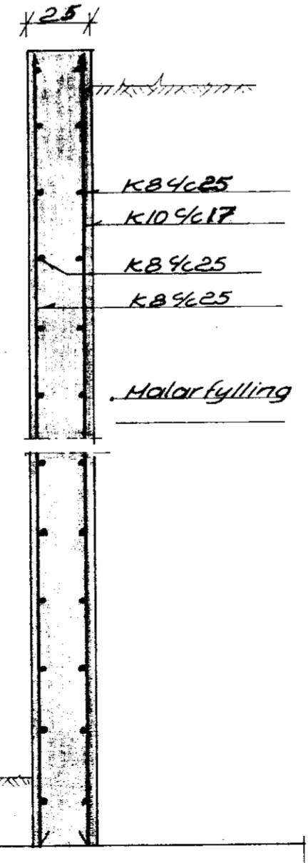
Snid D-D M1:20
