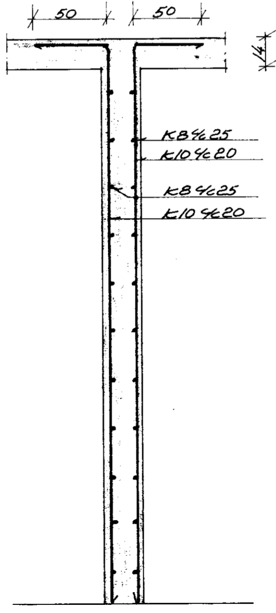
Snid C-C M1:20
