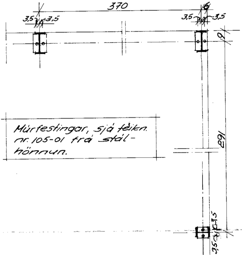
Murfestingar M1:20
