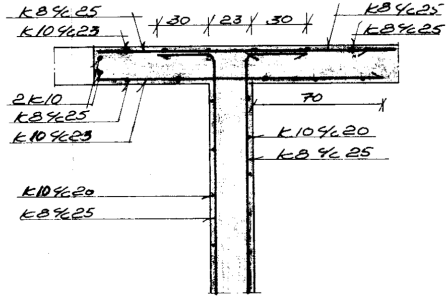
Larett snid i vegg M1:20
