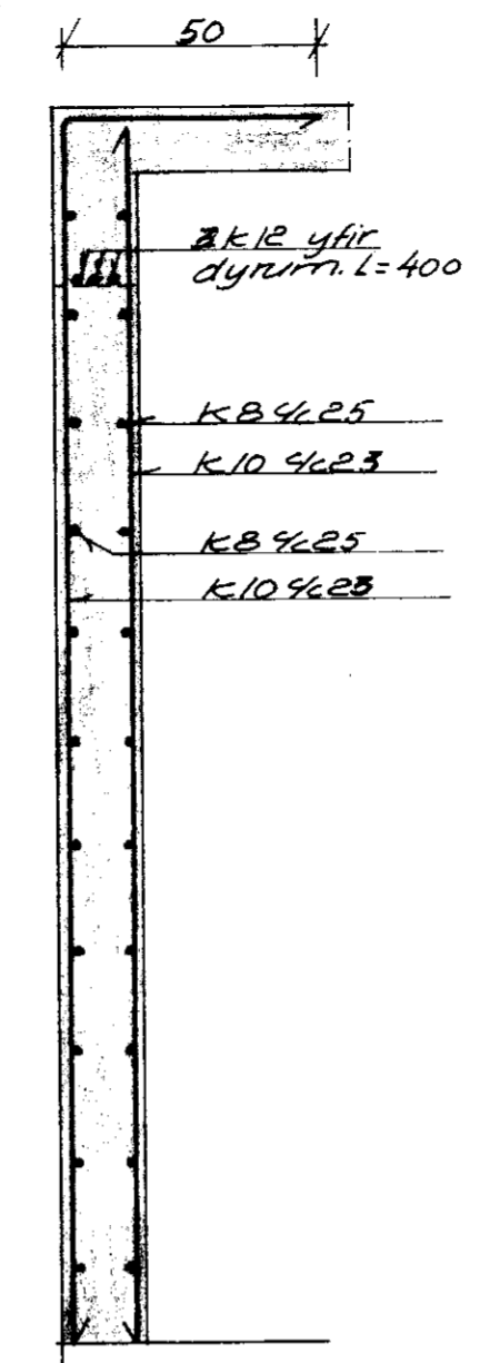
Snid B-B M1:20
