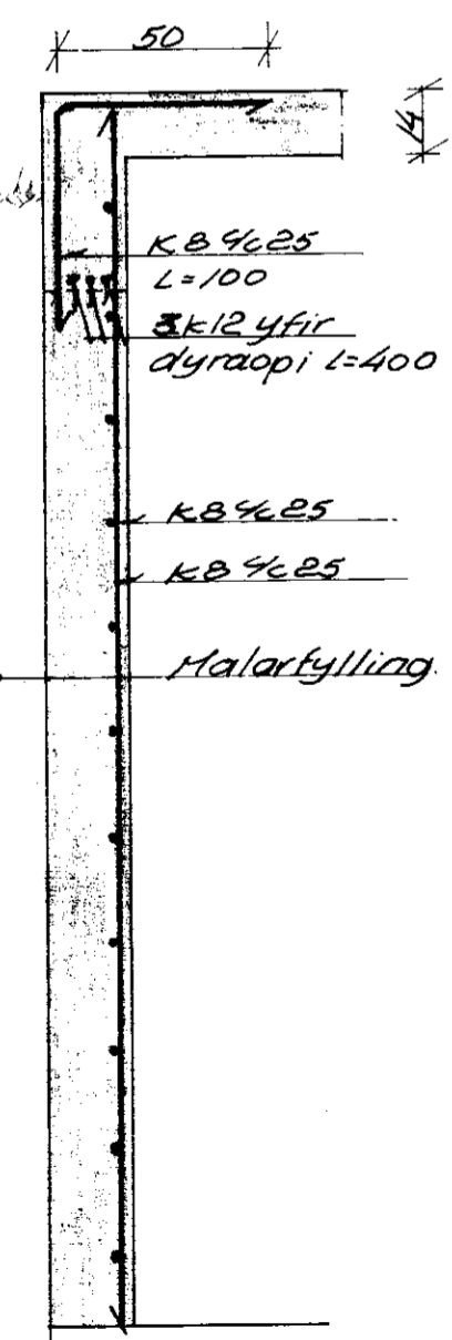
Snid E-E M1:20
