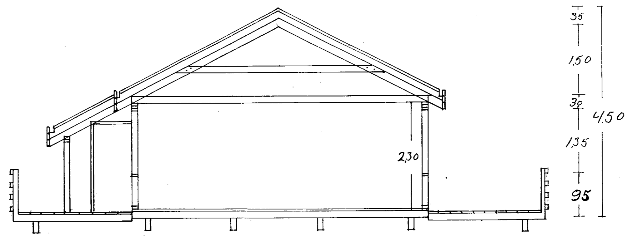
Snið A-A
