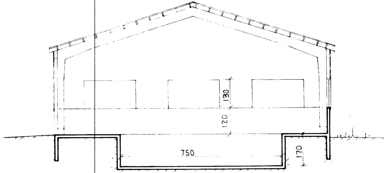
SNIÐ A-A 1:100
