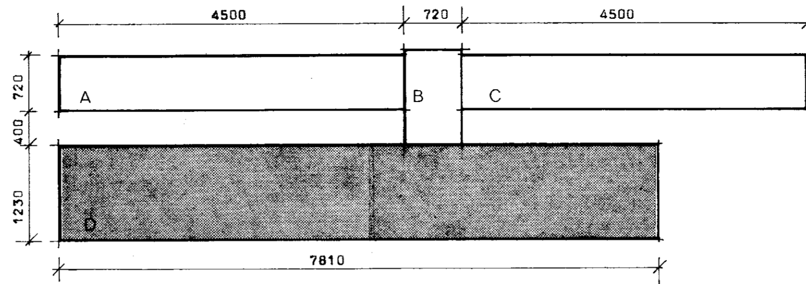
AFSTÖÐMYND. M 1:500
