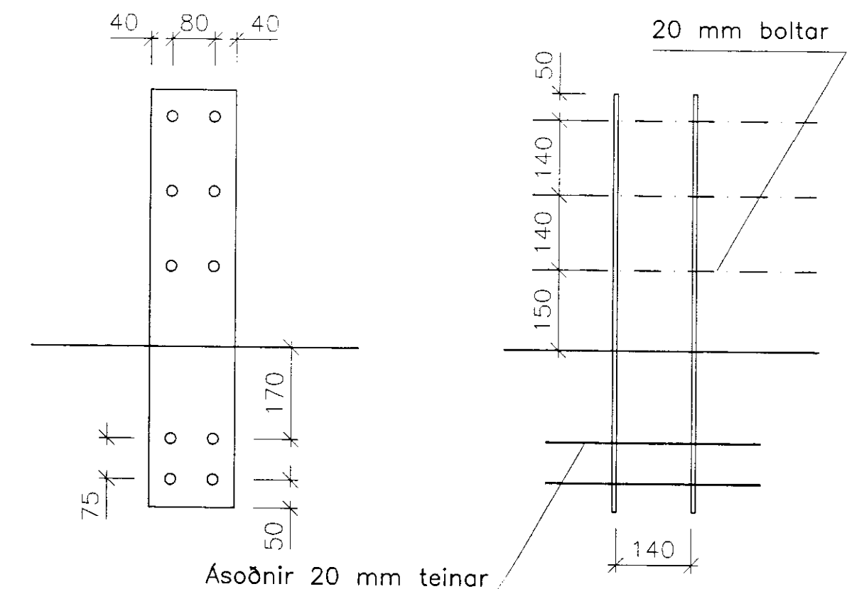
FESTING F2 1:10
