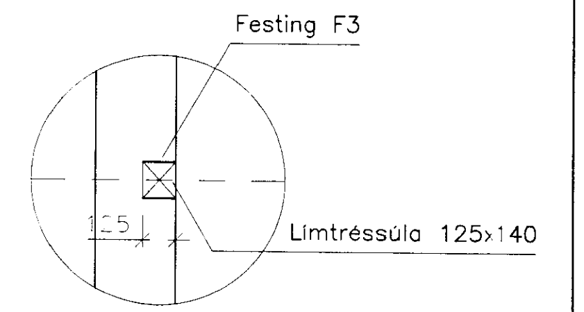
SÉRMYND 1 1:20
