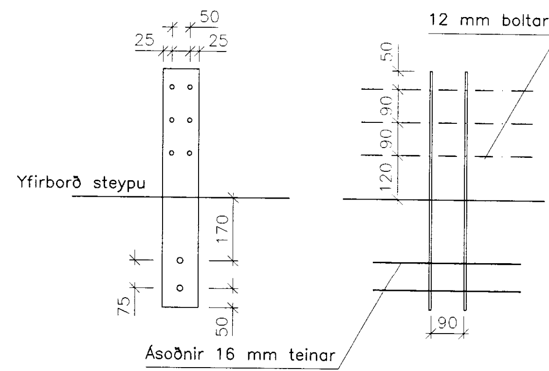
FESTING F1 1:10
