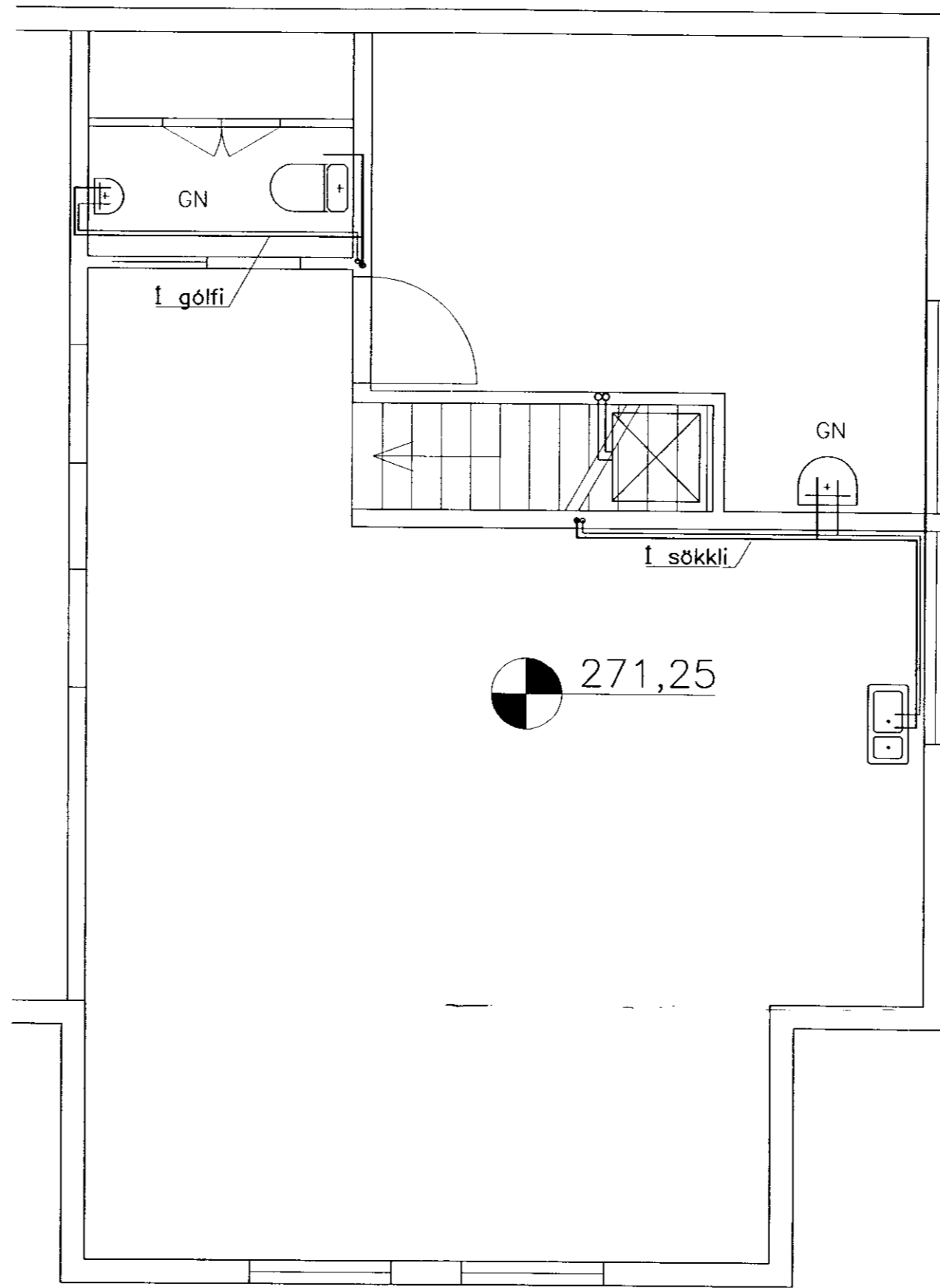
GRUNNMYND 2. HÆÐ 1:50
