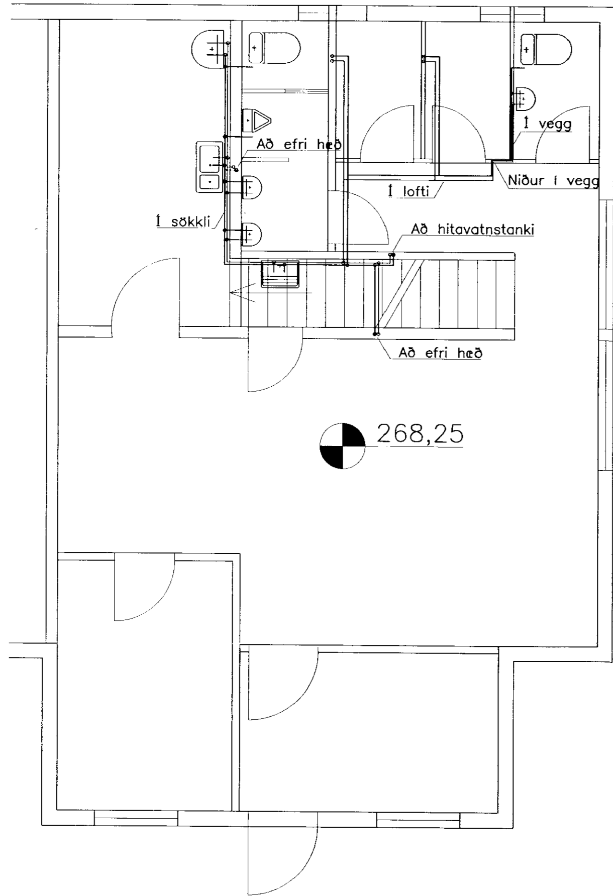
GRUNNMYND 1. HÆÐ 1:50
