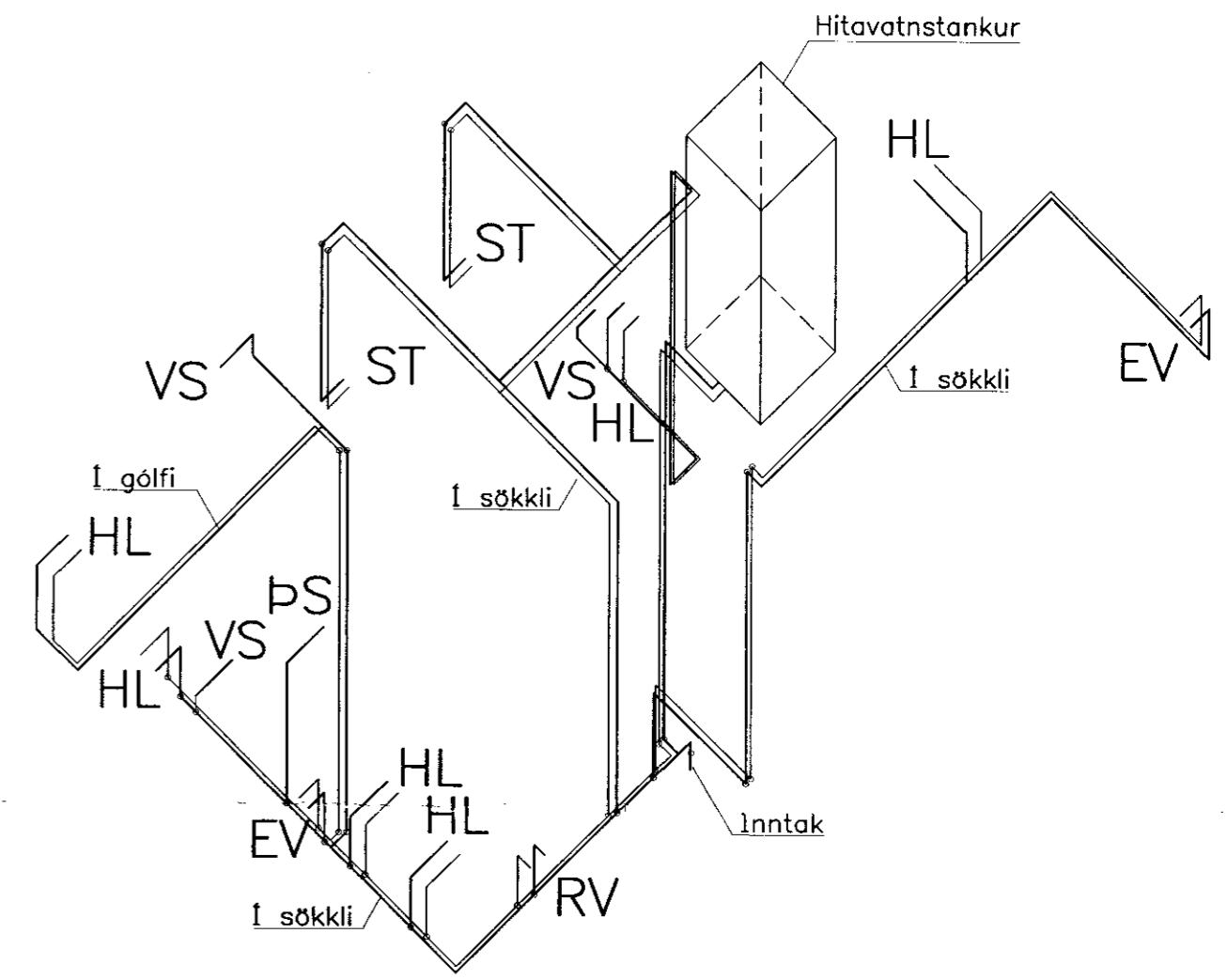
RÚMMYND 1:50
