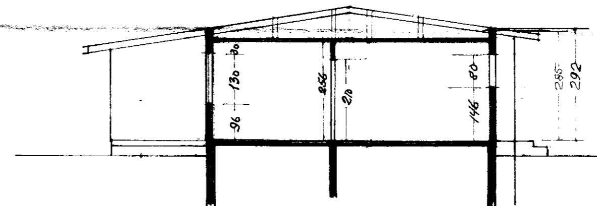
Skurður a-b
