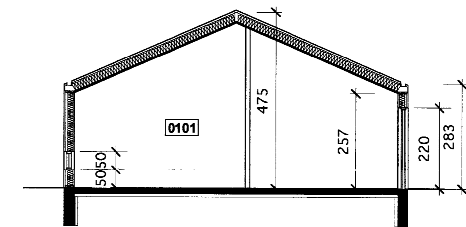
SNÍÐ A-A
