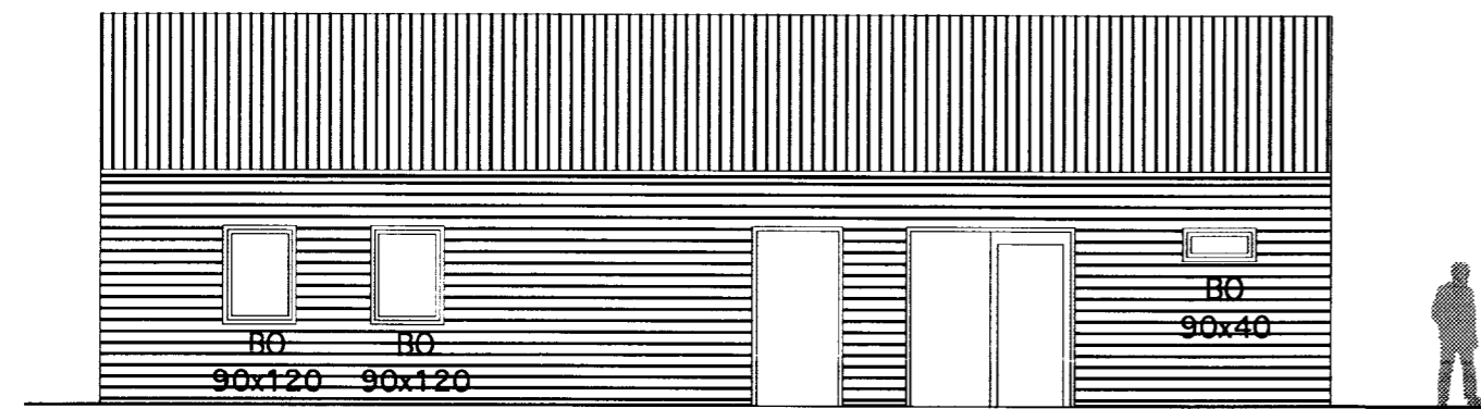
ÚTLIT - NORÐUR
