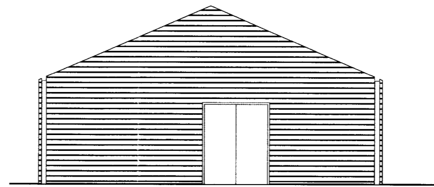
ÚTLIT - AUSTUR
