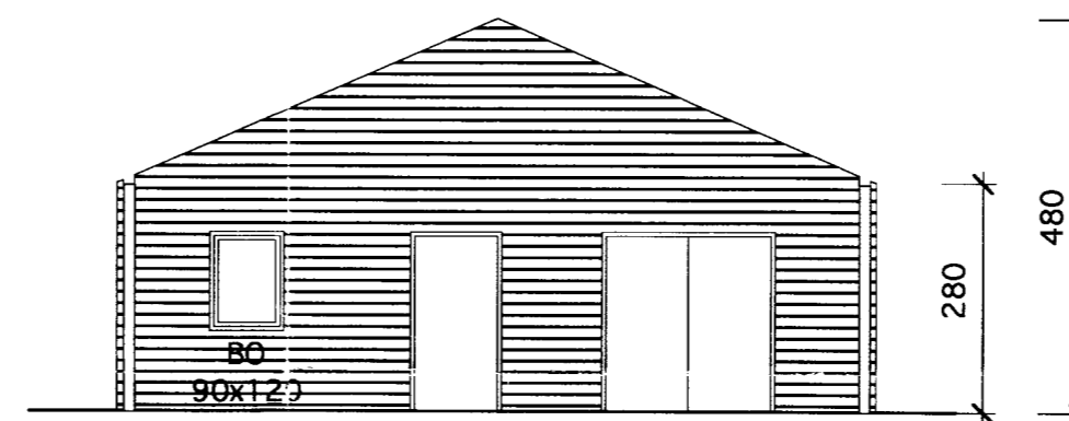
ÚTLIT - VESTUR
