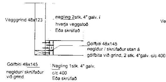
SNIÐ D-D 1:20
