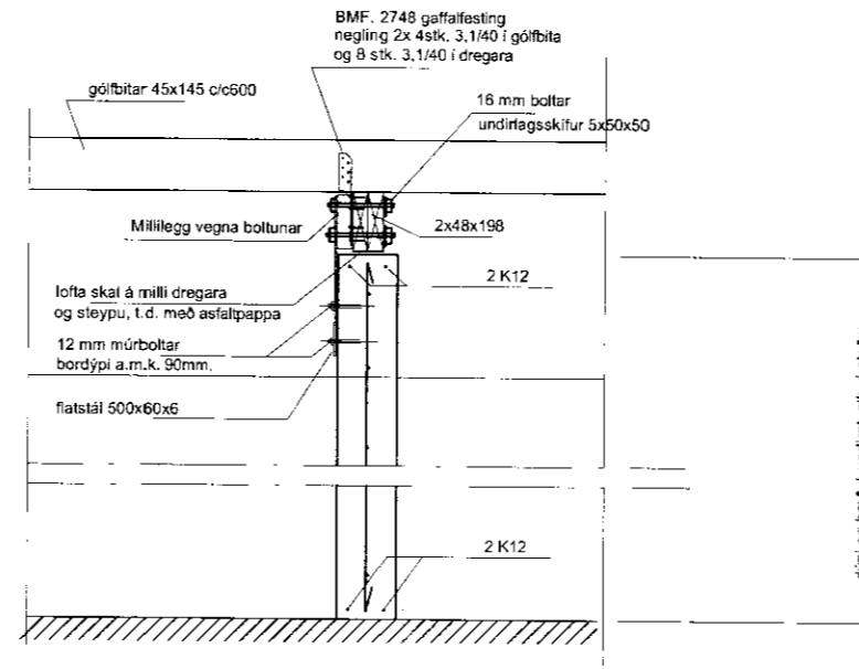
SNIÐ B-B 1:20
