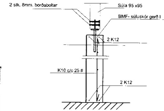
SNIÐ C-C 1:20
