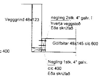
SNIÐ E-E 1:20
