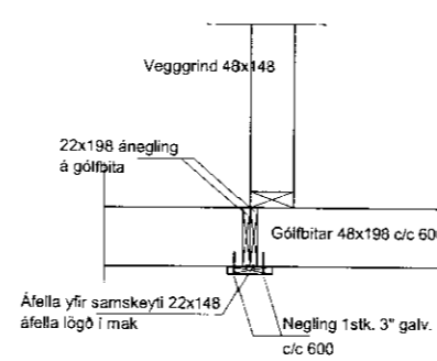
SNIÐ G-G 1:20
