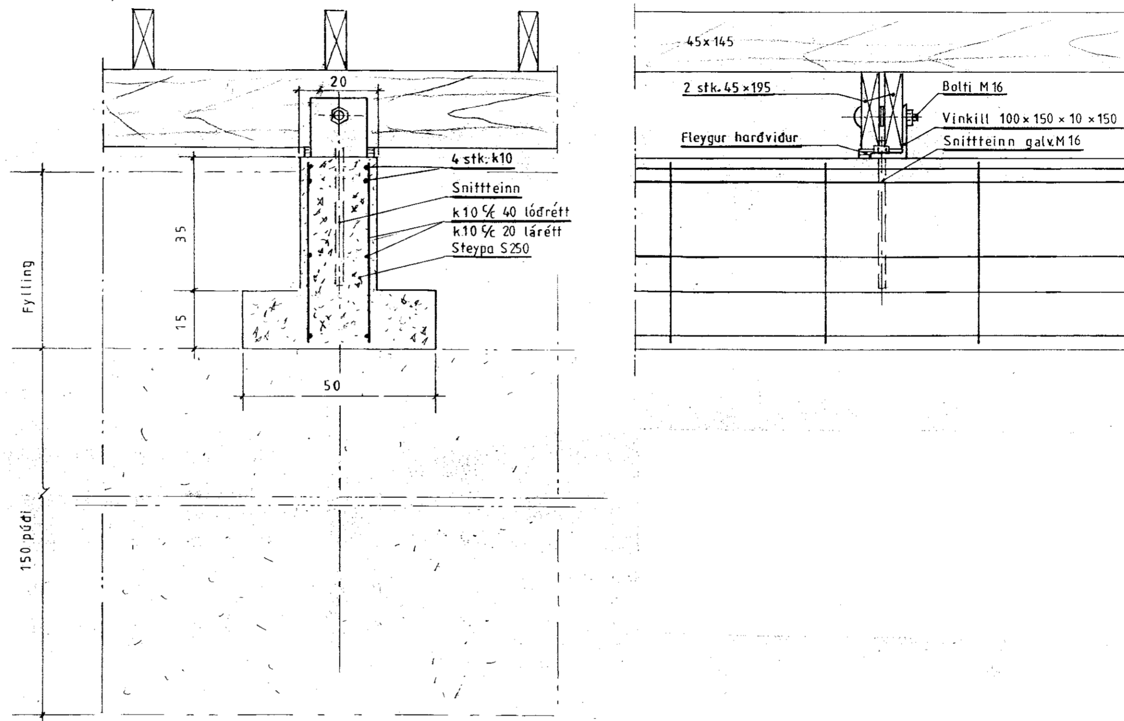
Snið A-A
