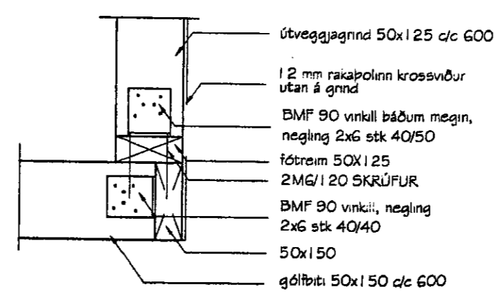
SNIÐ 3-3 mkv. 1:10
