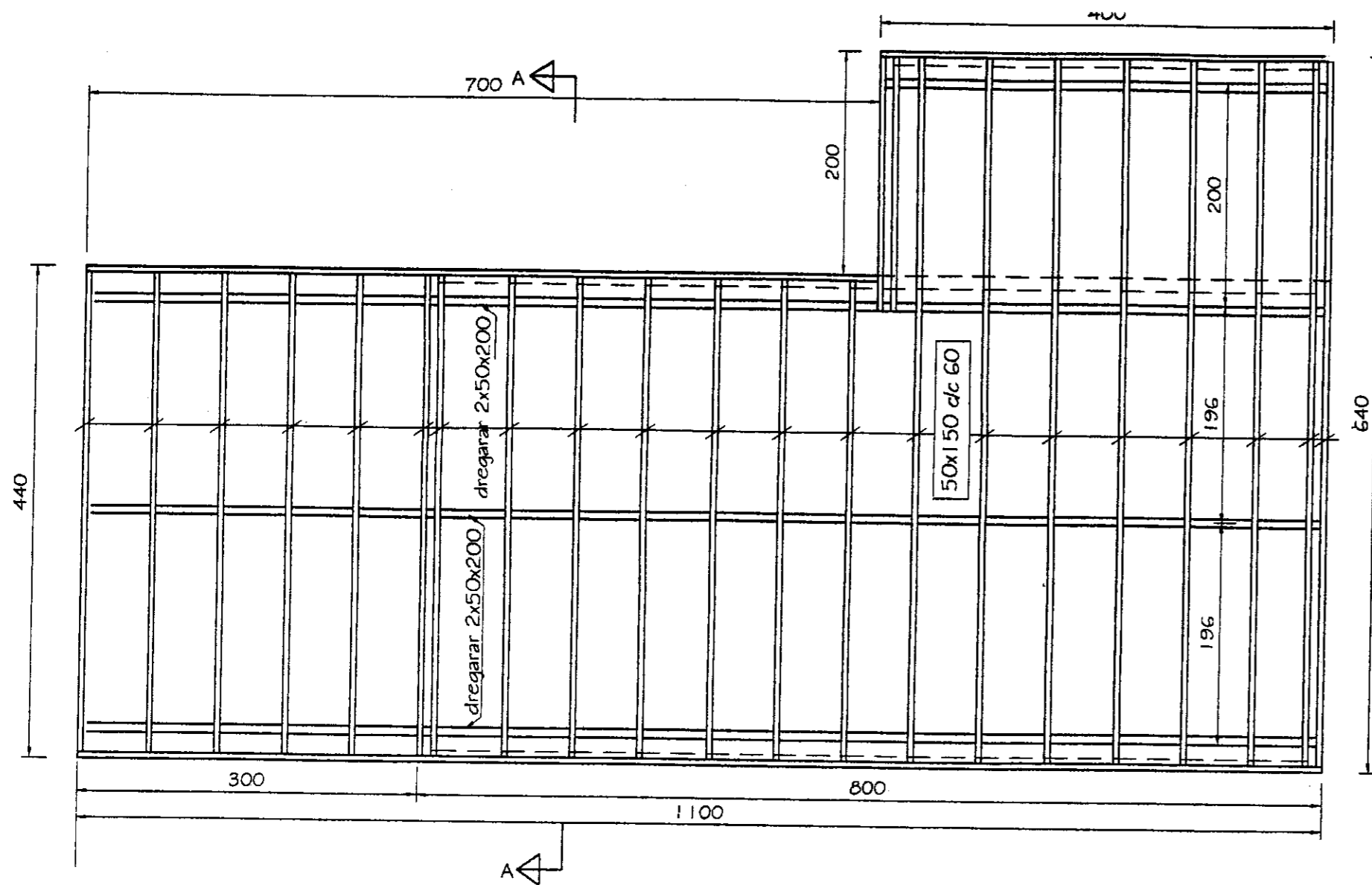
DREGARAR OG GÓLFBITAR GRUNNMYND mkv. 1:50
