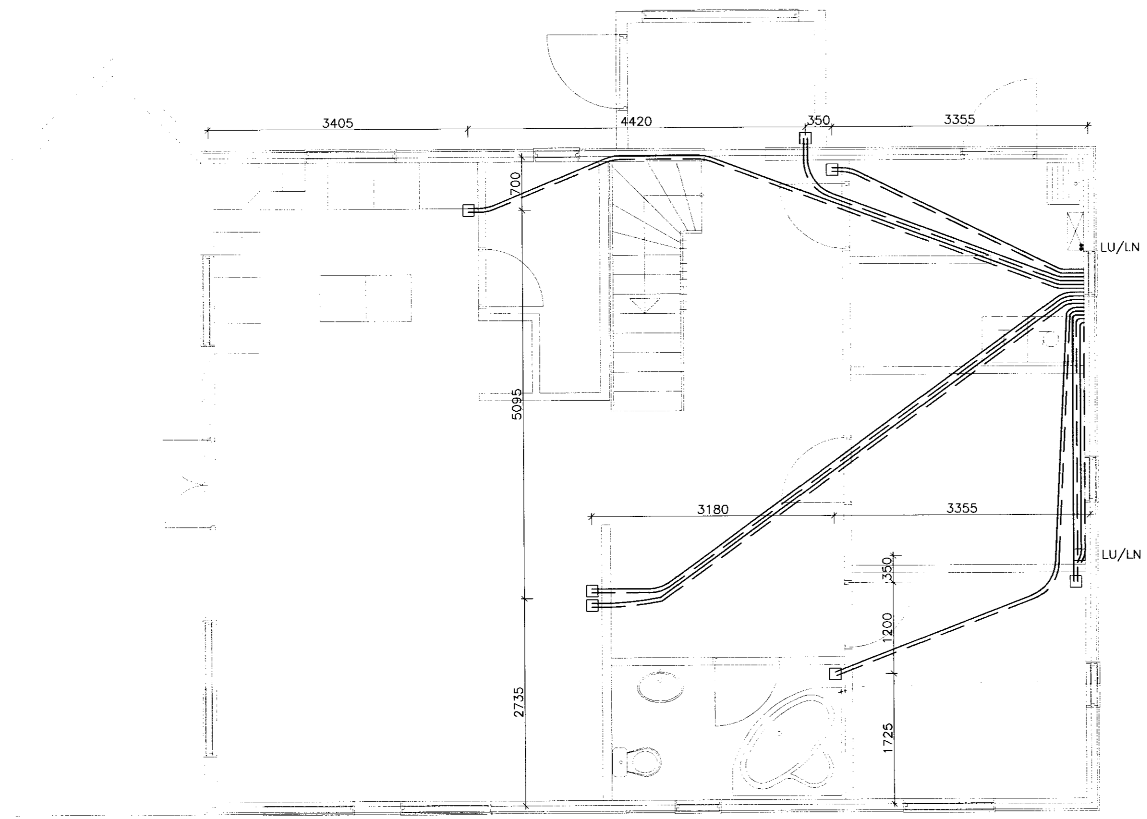
1. HÆÐ GRUNNMYND GÓLFGEISLALAGNA 1:50
