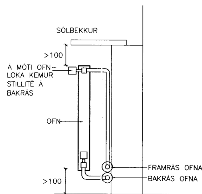
SNID Í VEGG Mkv. 1:10
