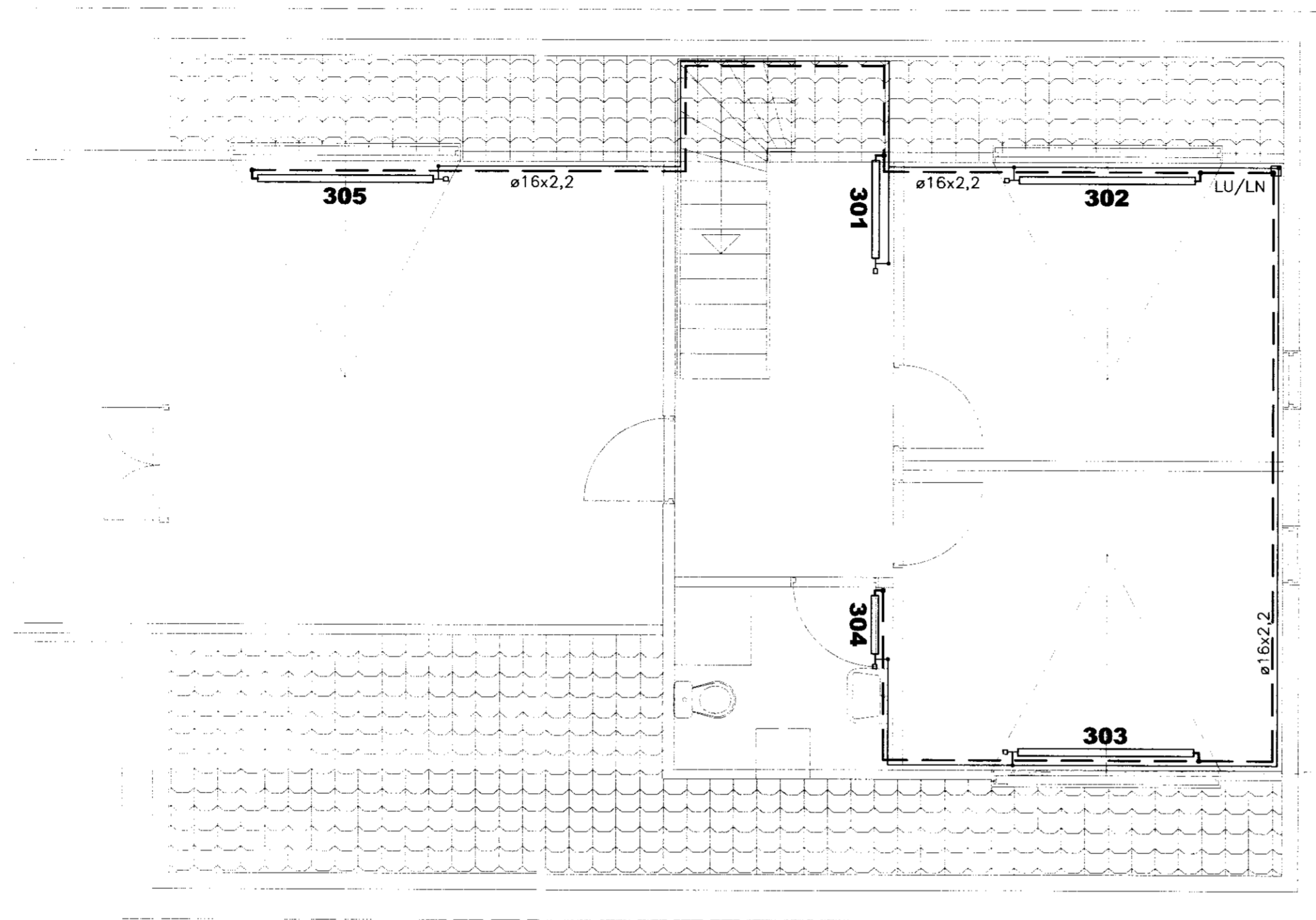
2. HÆÐ GRUNNMYND OFNALAGNA 1:50
