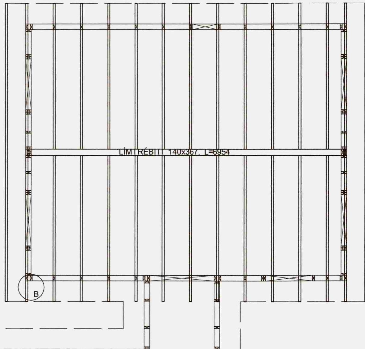
SPERRUPLAN, MKV. 1:50
