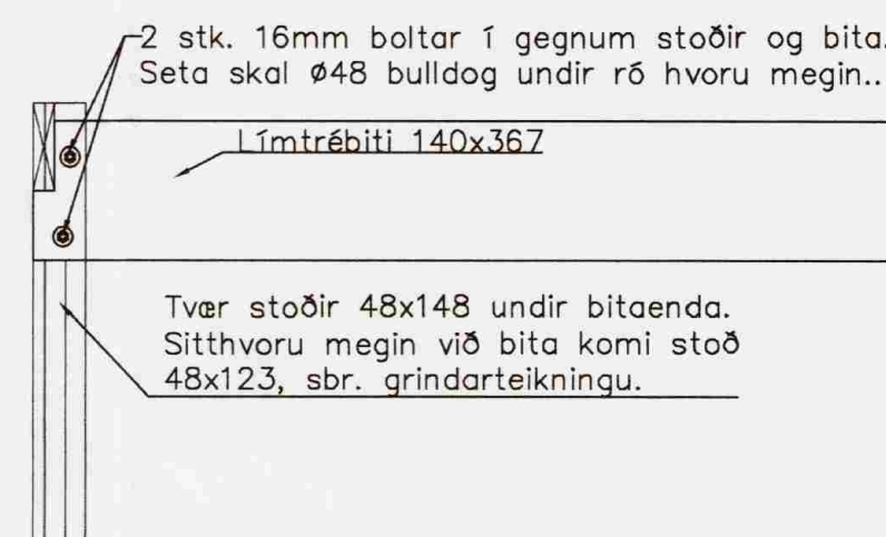
DEILI D, FESTING BITA VIÐ ÚTVEGG, MKV. 1:20
