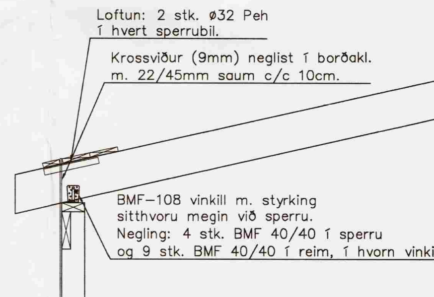
DEILI B, FESTING SPERRA VIÐ ÚTVEGG, MKV. 1:20
