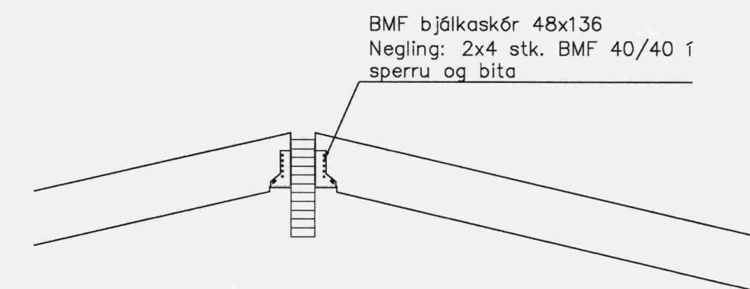
DEILI C, FESTING SPERRA VIÐ MÆNISBITA, MKV. 1:20
