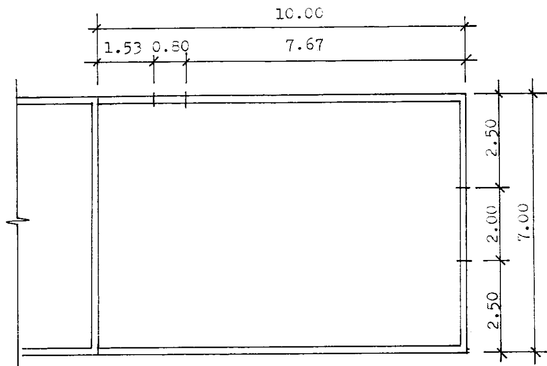
GRUNNMÝND 1:100
