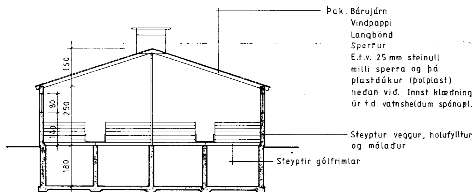
Snid A-A (Sjá bl.nr.2) M = 1:100
