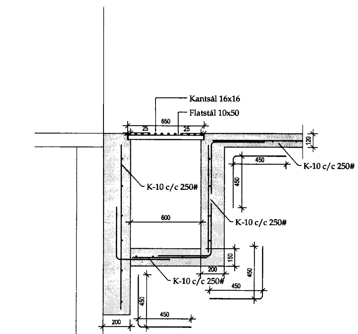
Snið D mk. 1:20
