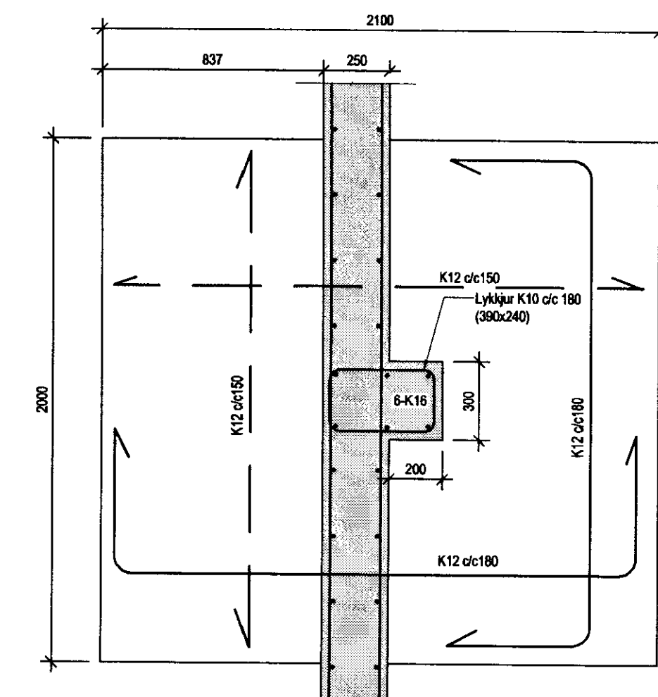
Snið A2 mk. 1:20
