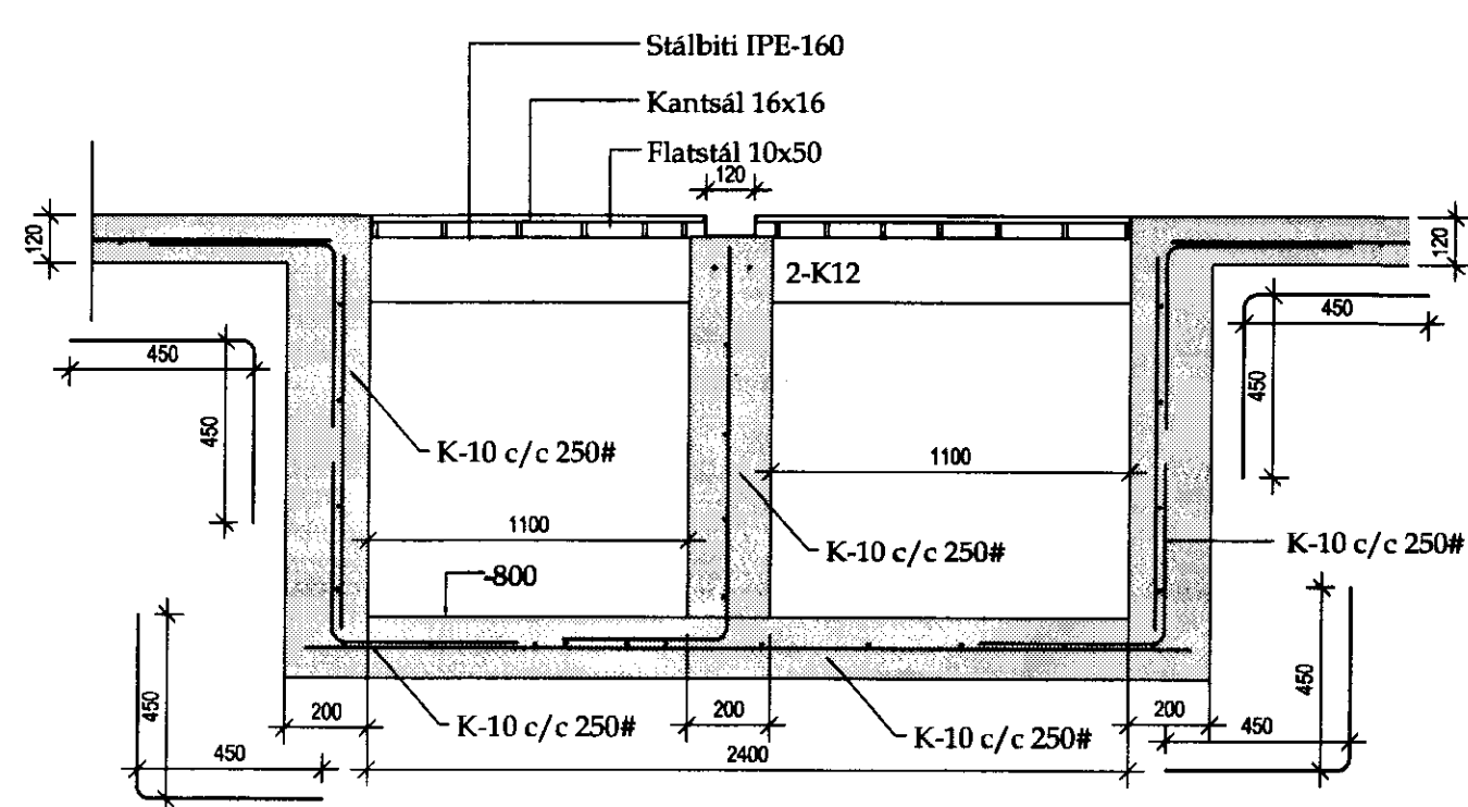
Snið B mk. 1:20
