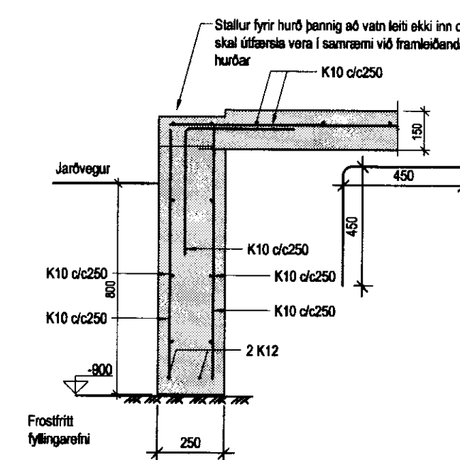
Snið A3 mk. 1:20
