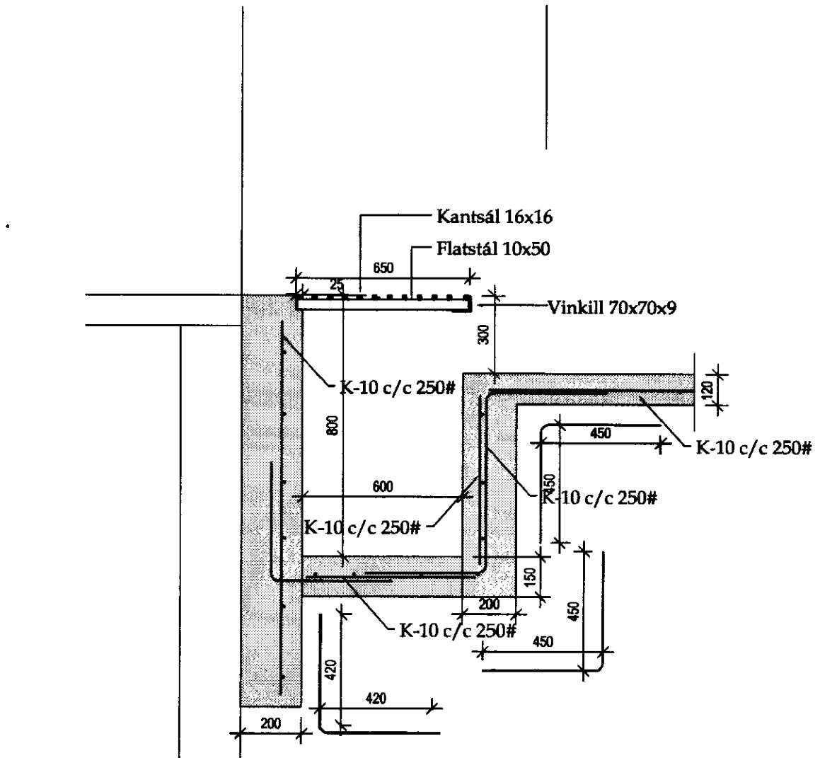
Snið D1 mk. 1:20
