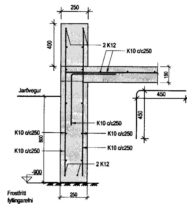
Snið A1 mk. 1:20
