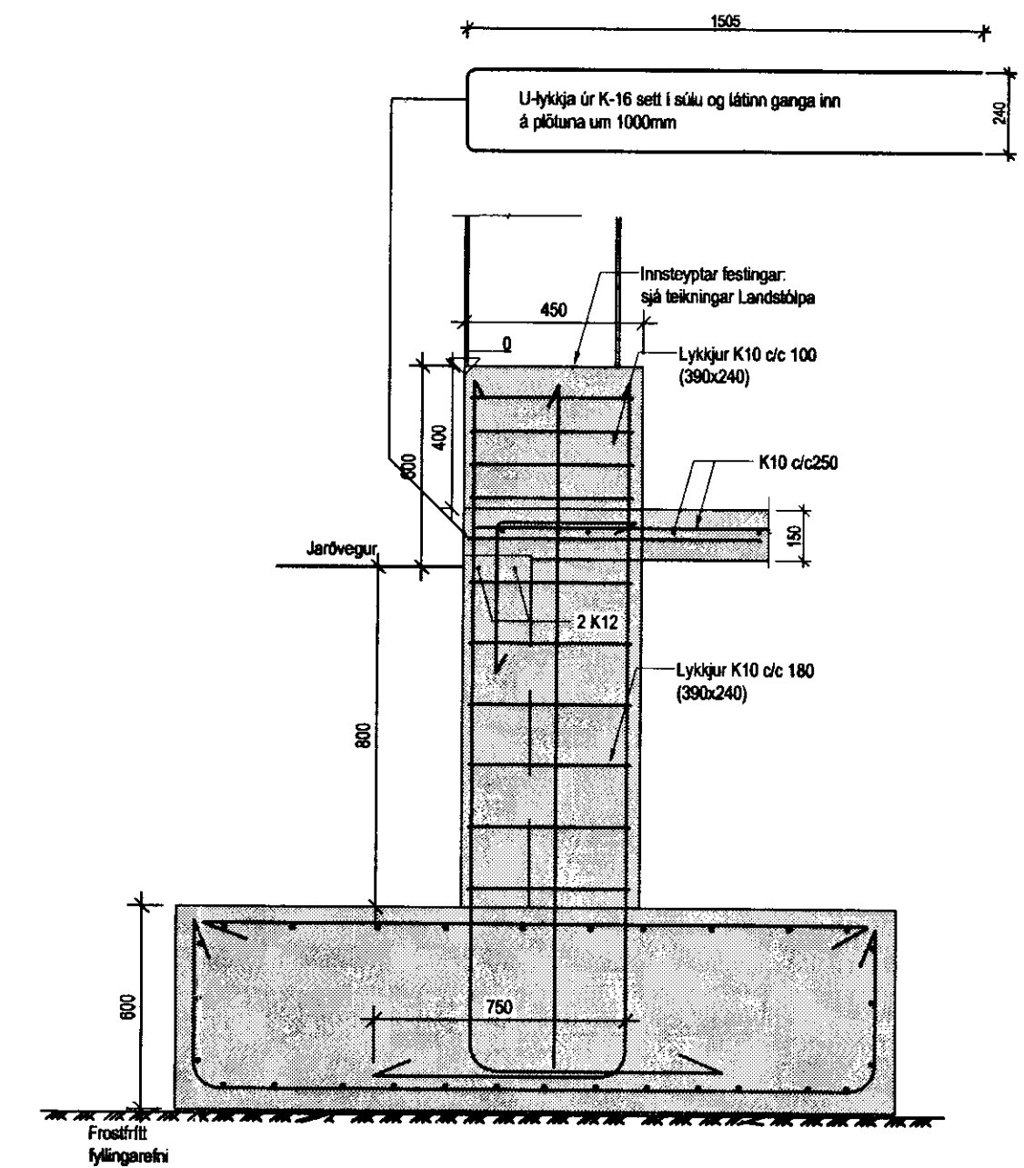
Snið A2 mk. 1:20
