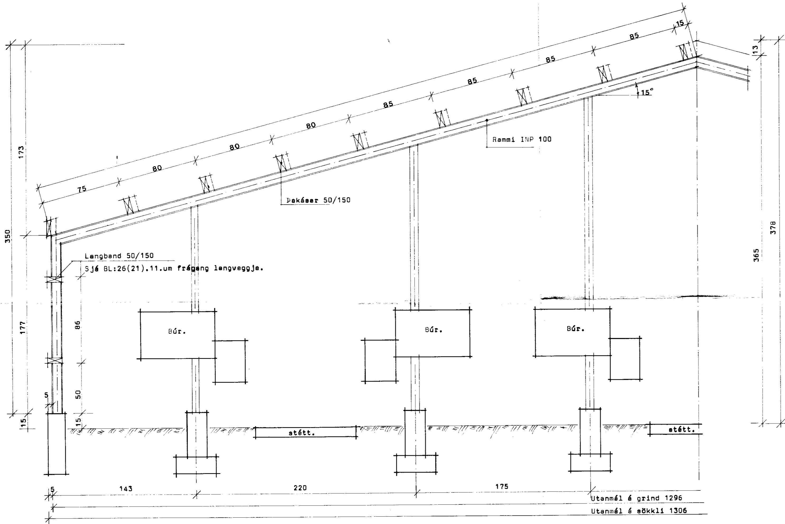
ÞVERSNIÐ (Hluti.) M 1:20 Staðsetning þakáæa & langbands.
