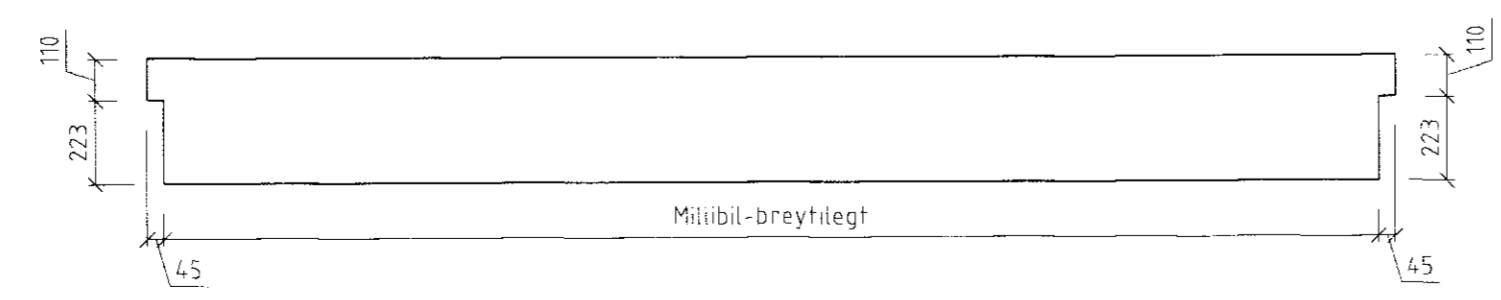
Endasögun á gluggabirum GB1-90x333-12 stk.
