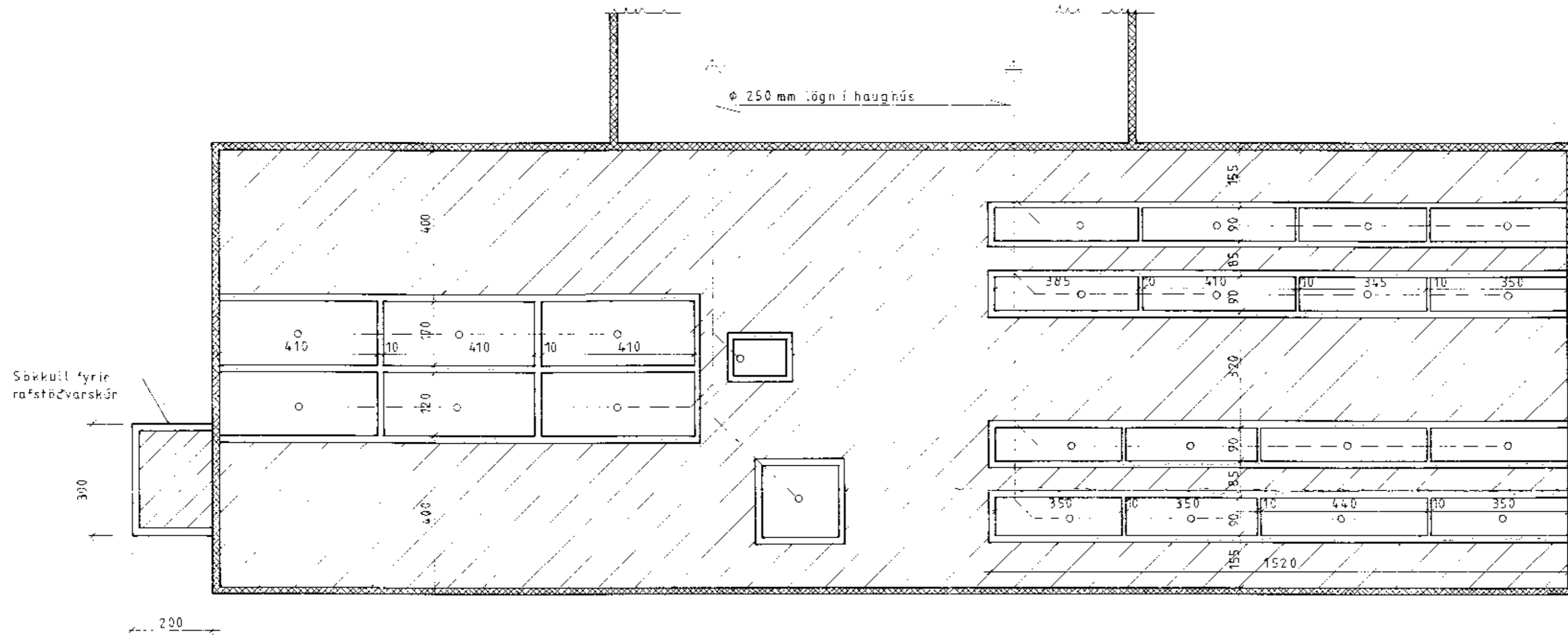
Flórar M = 1:100
