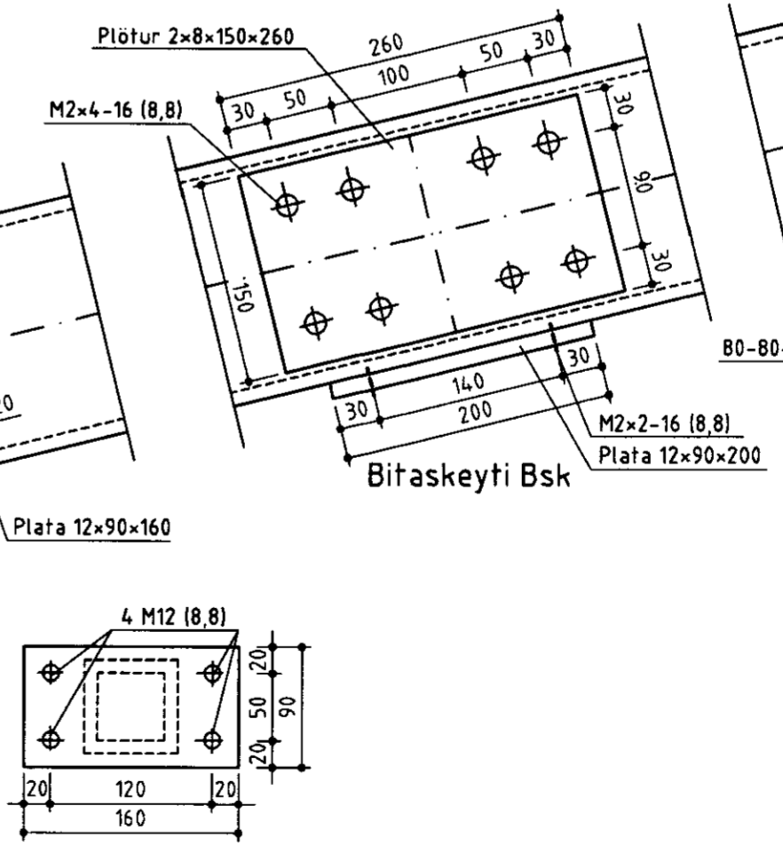
Deili Mkv. 1:5
