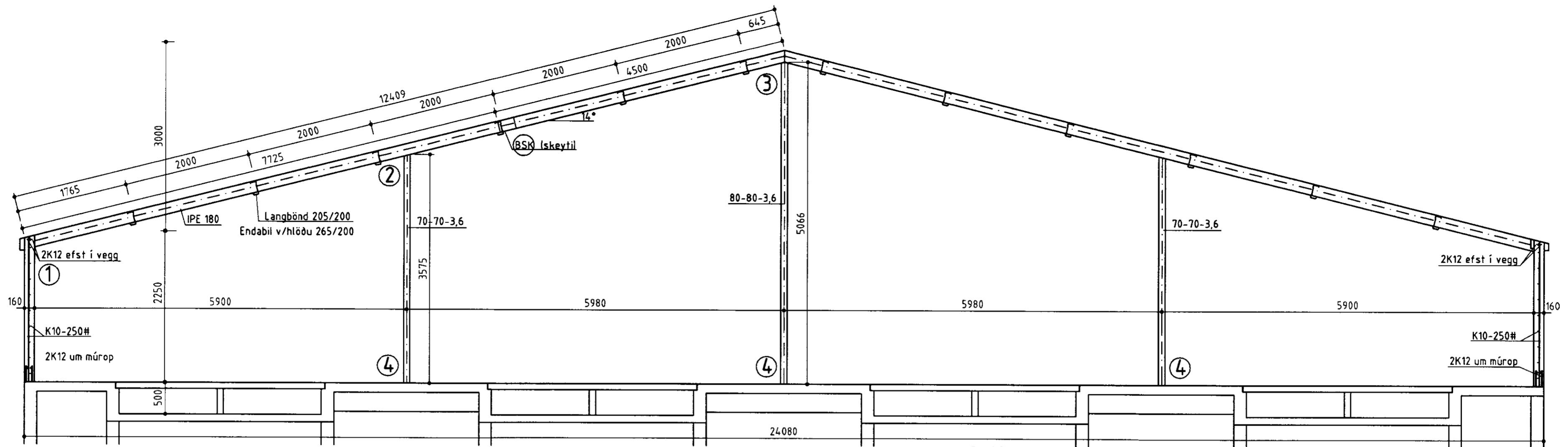
Snið Mkv. 1:50
