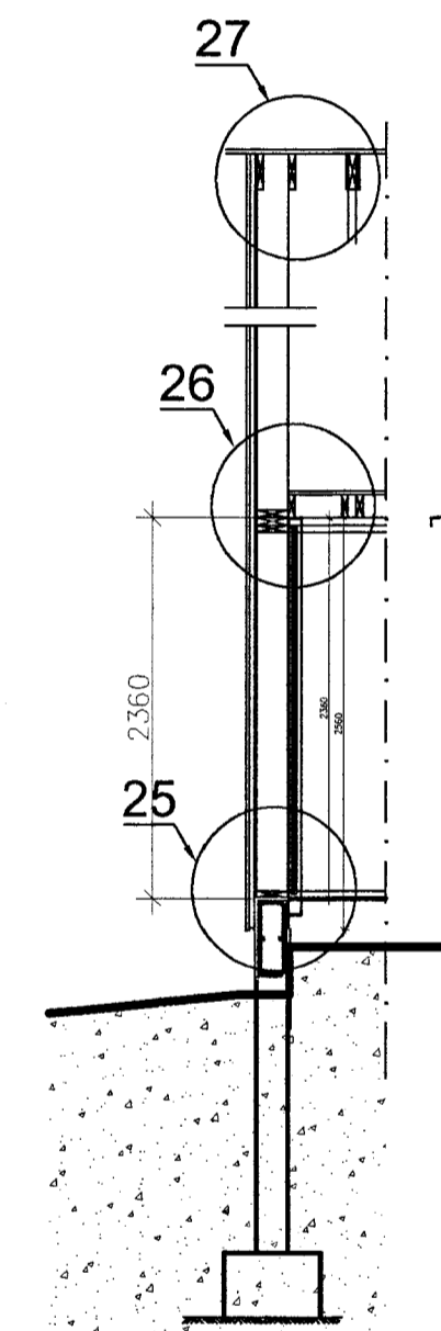
Snið B 1/50
