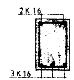
C-C M=1:20
