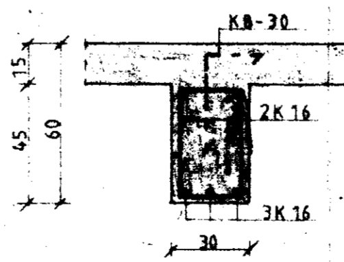
SNID A-A M=1:20
