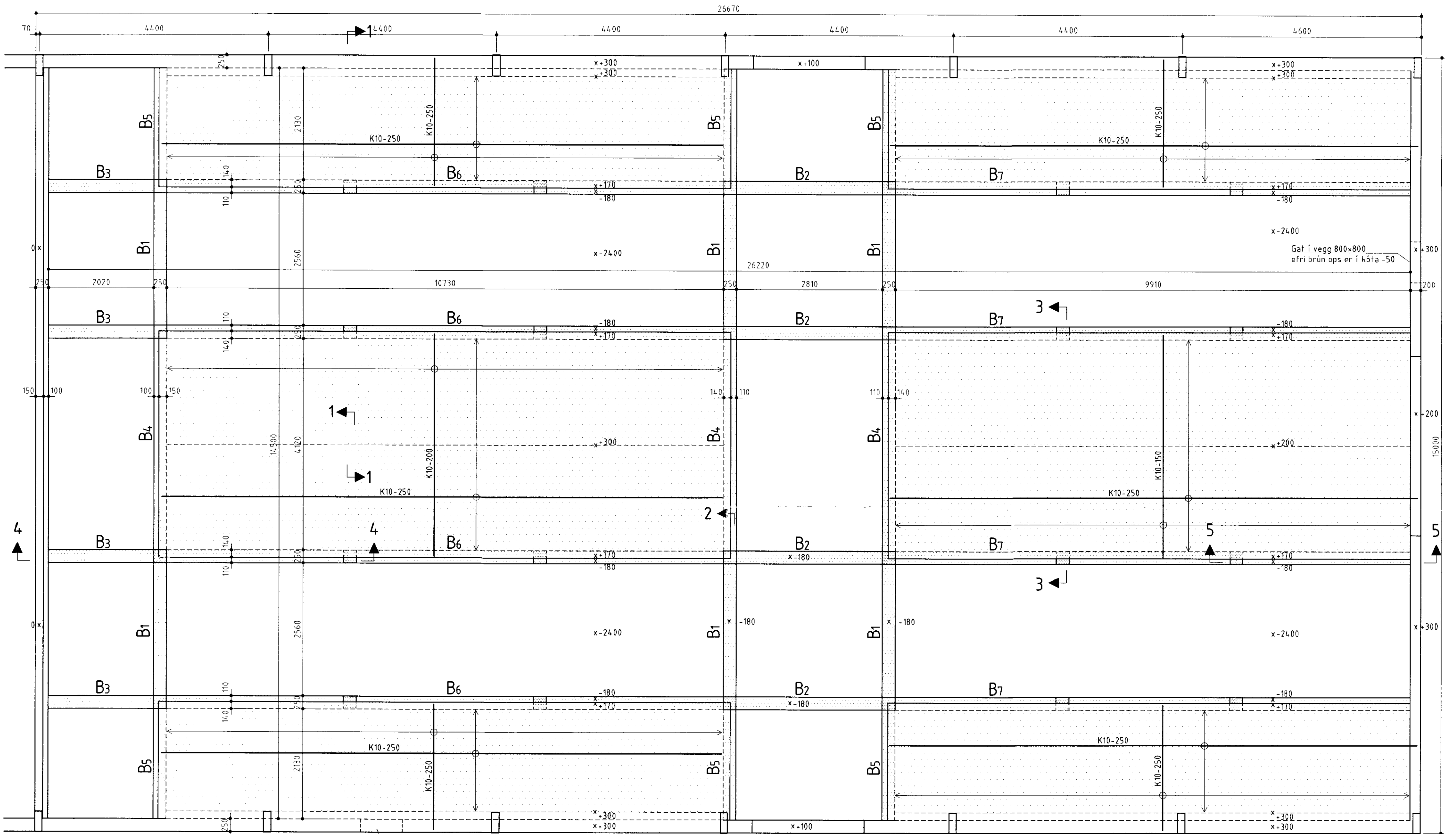
Gólfplata Mkv. 1:50
