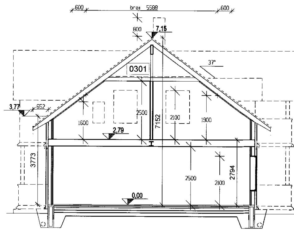
Snið A-A
