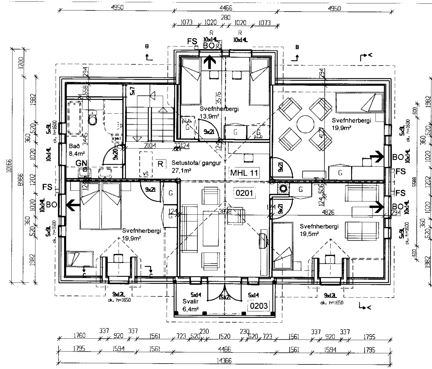
2. hæð
