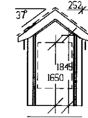
Snið C-C
