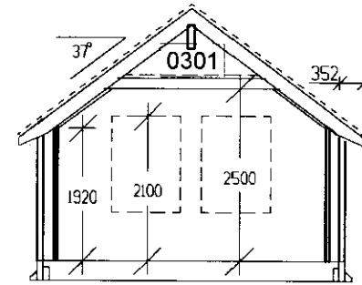
Snið B-B
