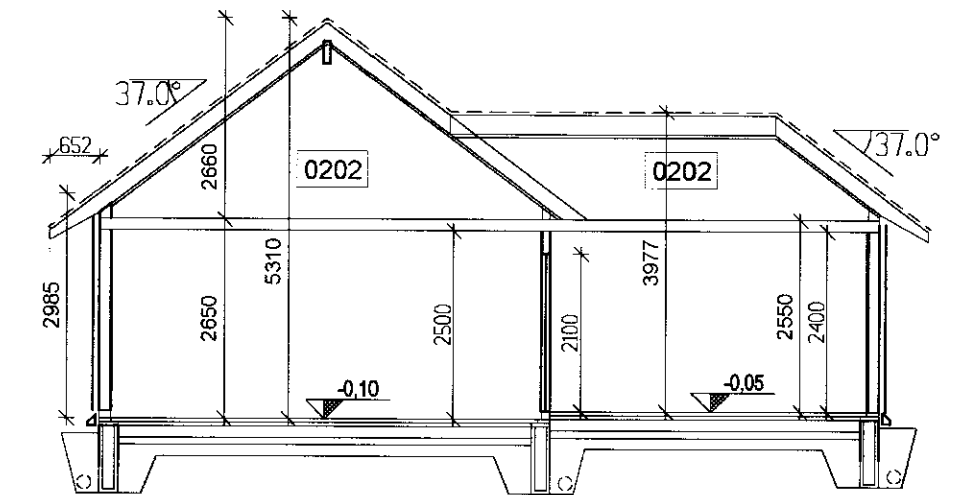
Snið D-D
