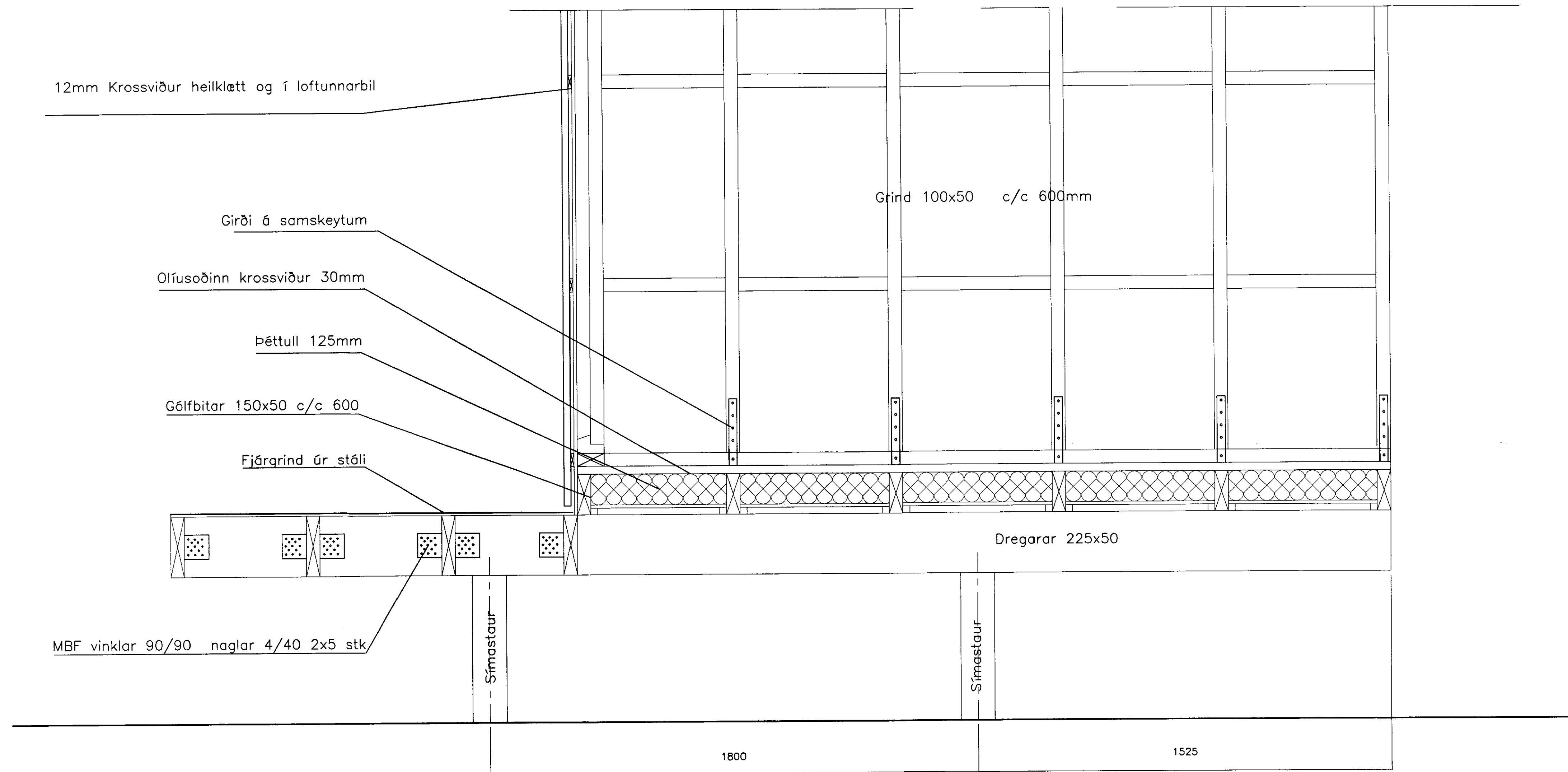
Snið A-A 1:20
