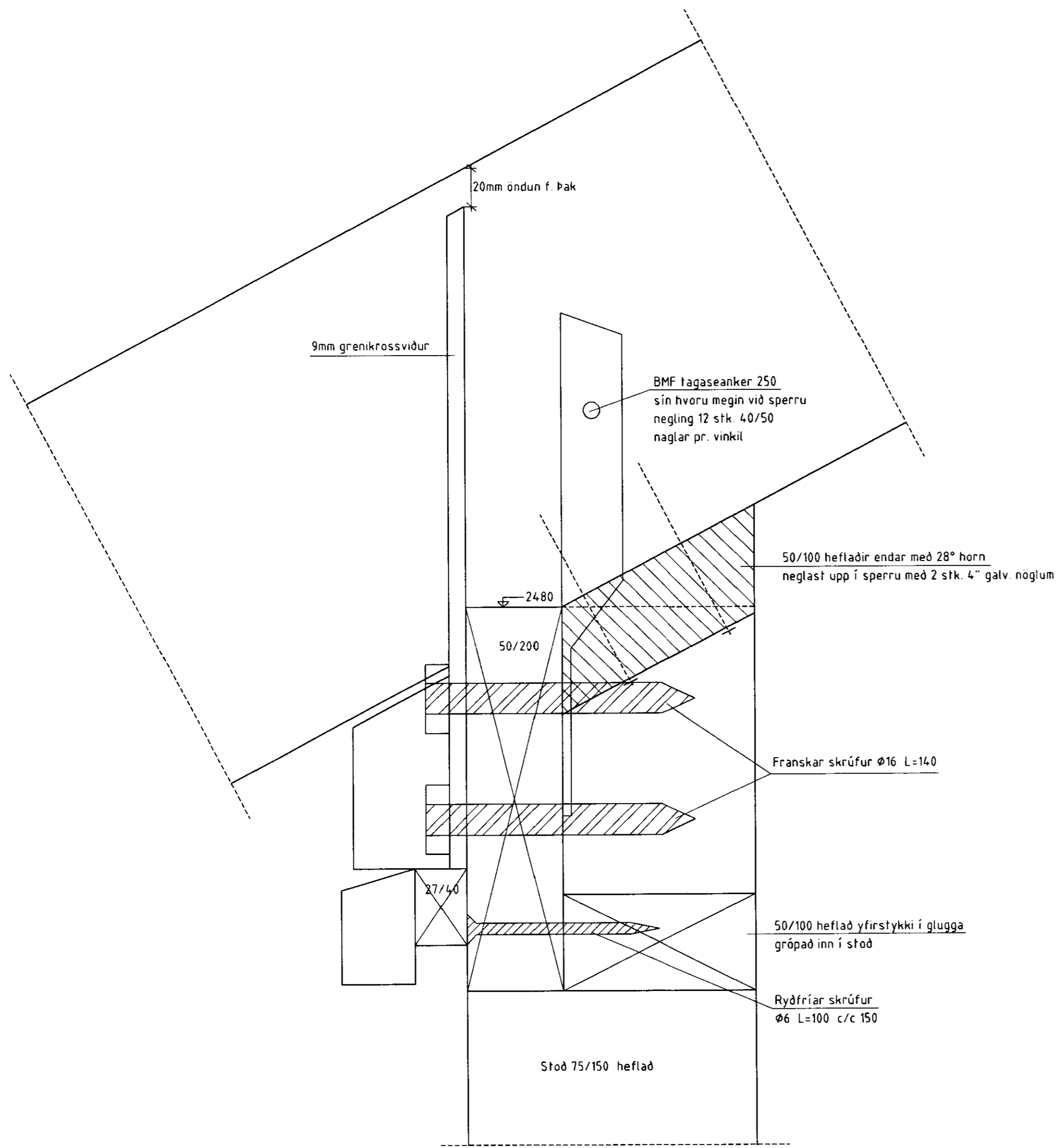
Snið D-D Mkv. 1:2
