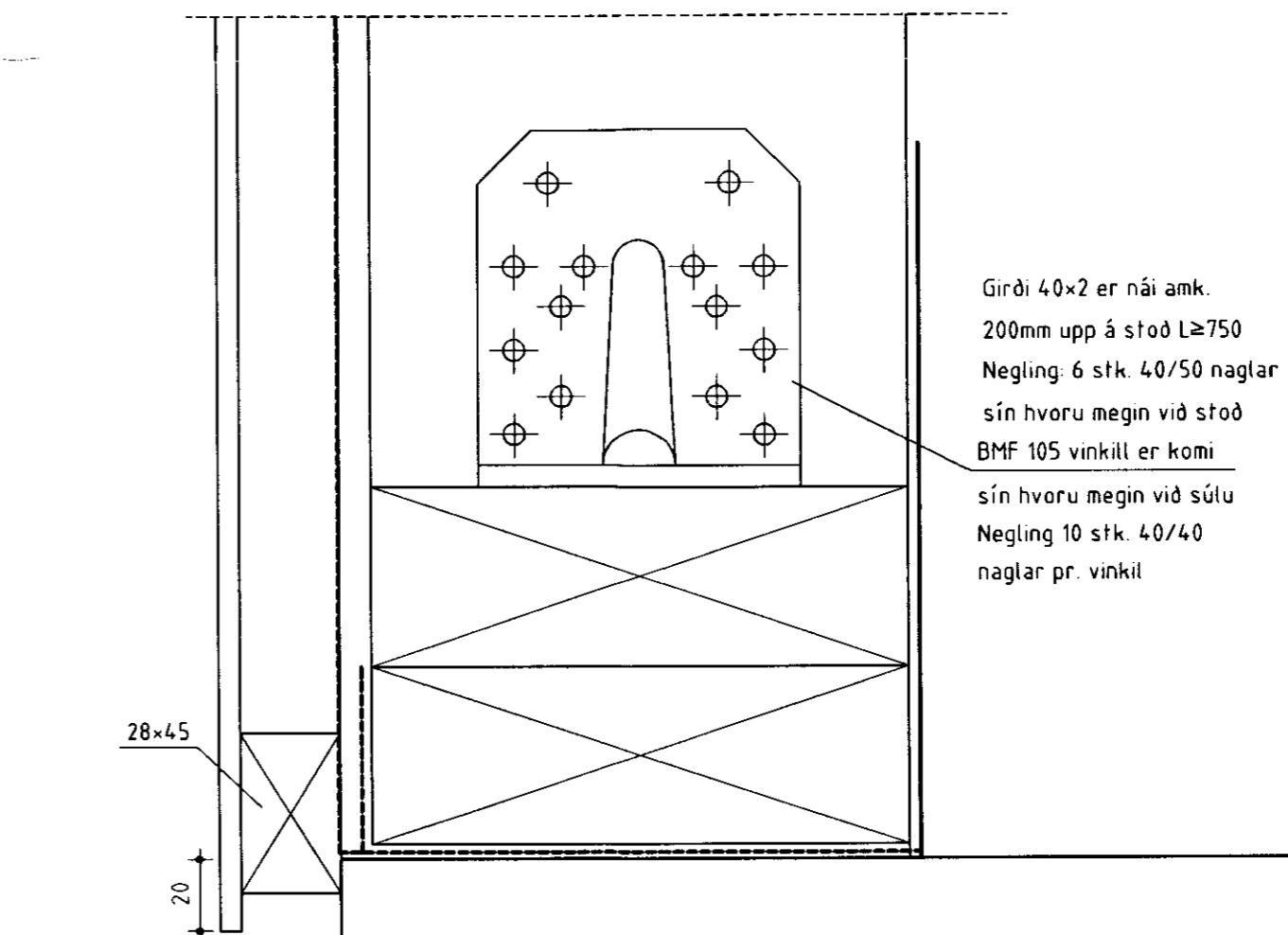
Sökkull Snið D-D Mkv. 1:2
