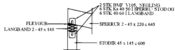
SNID A-A 1:20
