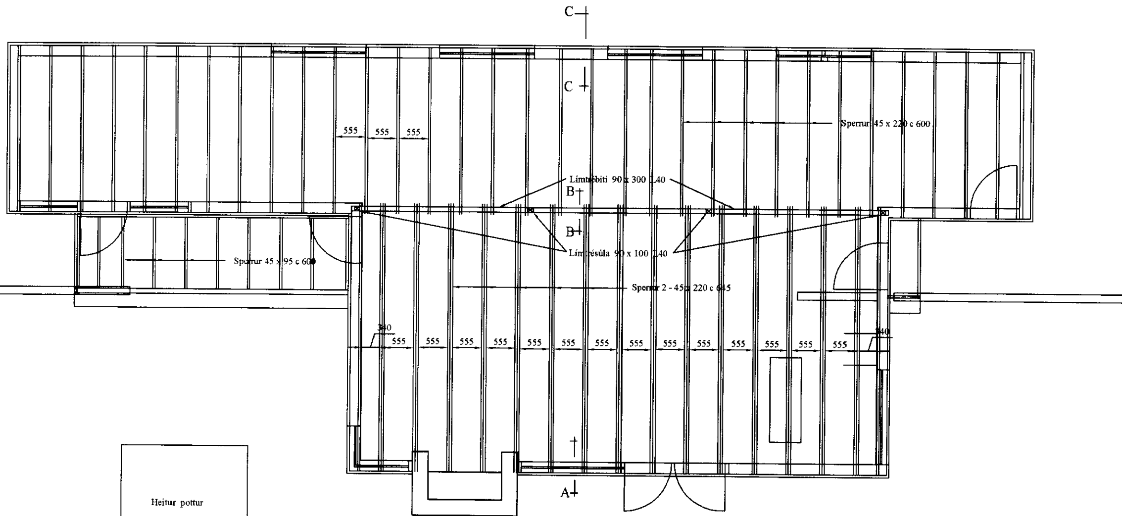
GRUNNMYND 1:50
