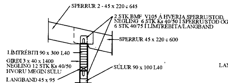
SNID B-B 1:20
