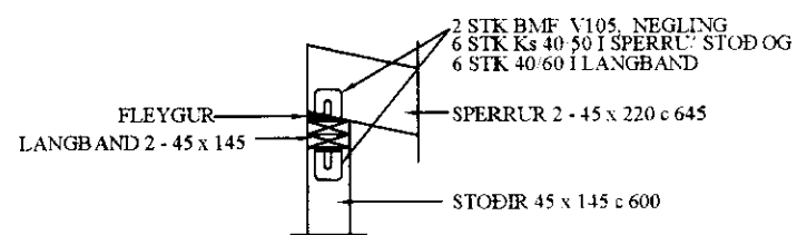
SNID A-A 1:20
