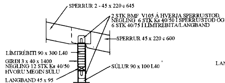
SNID B-B 1:20
