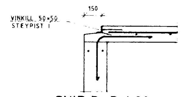
SNID B-B 1:20
