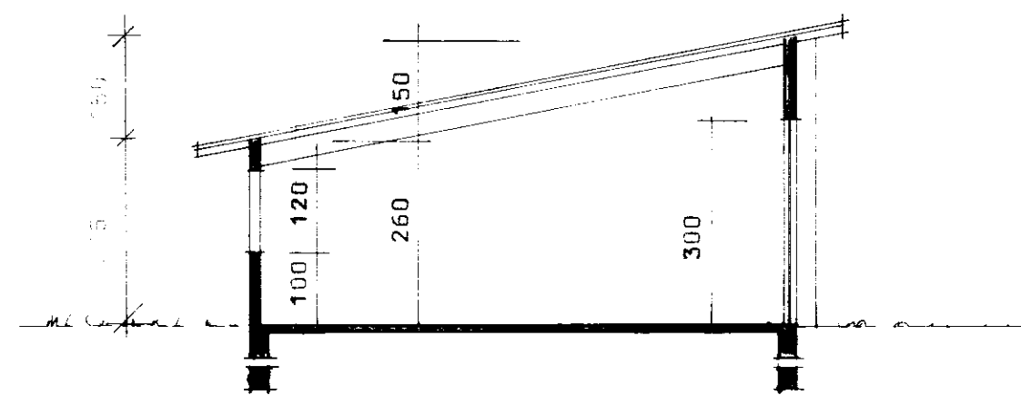
Snið a-a
