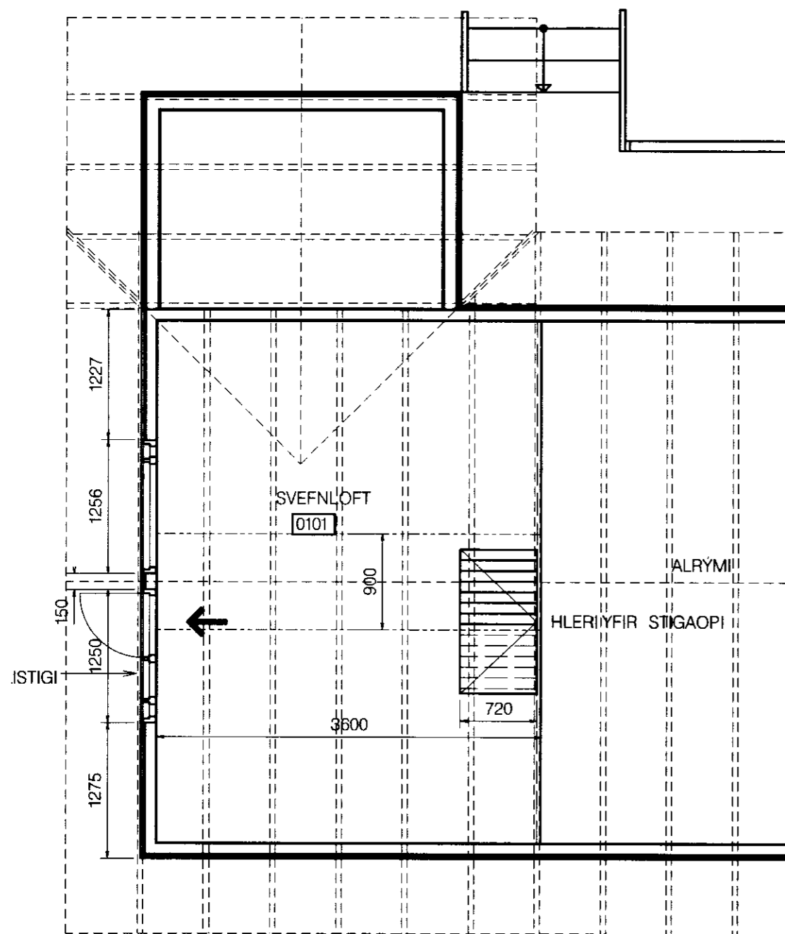
GRUNNMYND SVEFNLOFT MKV. 1:50
