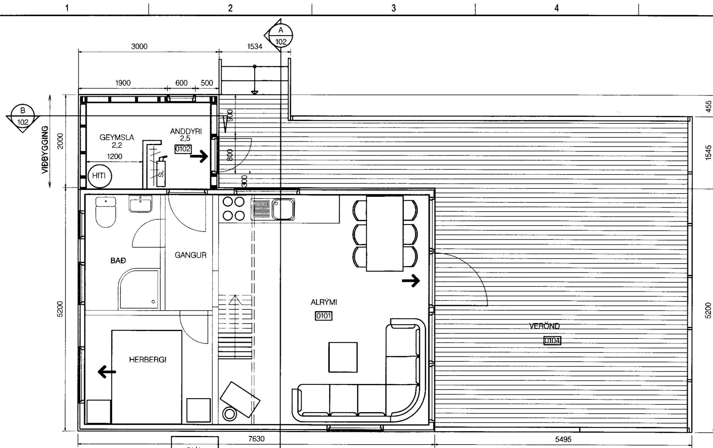
GRUNNMYND MKV. 1:50
