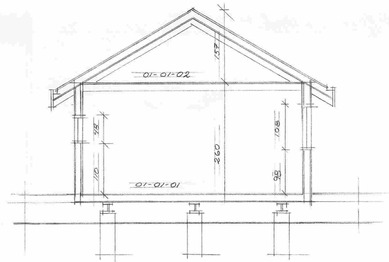
SNÍÐ R-A Í NUN. HÚS M=1:50
