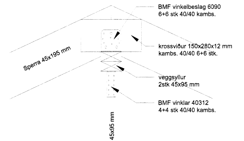
SNIÐ N-N (gestahús) sperrur á burðarvegg í mæni
