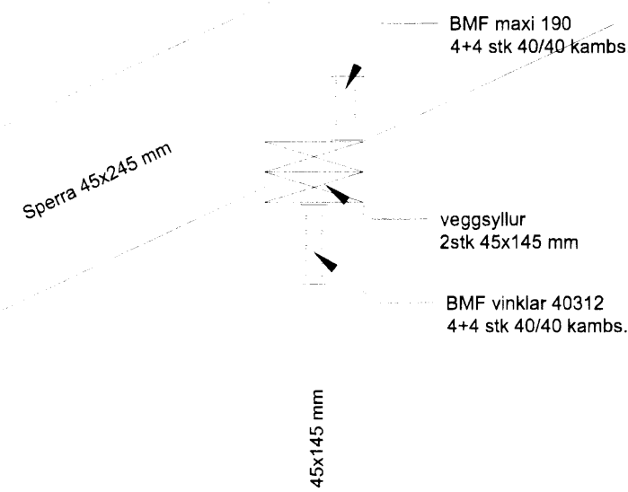
SNIÐ I-I (aðalhús) sperrur við útv.
