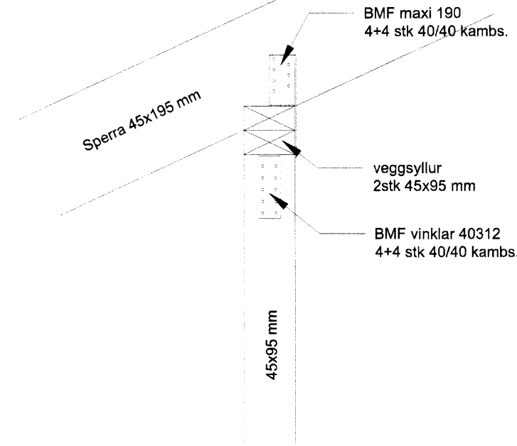
SNIÐ M-M (gestahús) sperrur við útv.
