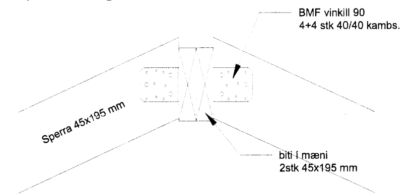
SNIÐ O-O (gestahús) sperrur og biti í mæni
