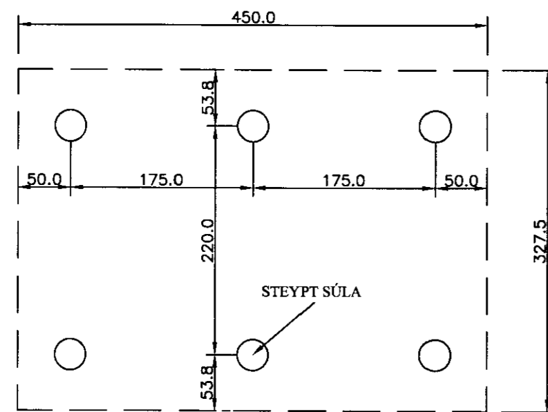
Grunnmynd steypar súlur
