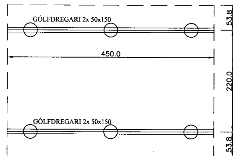
Grunnmynd dregarar
