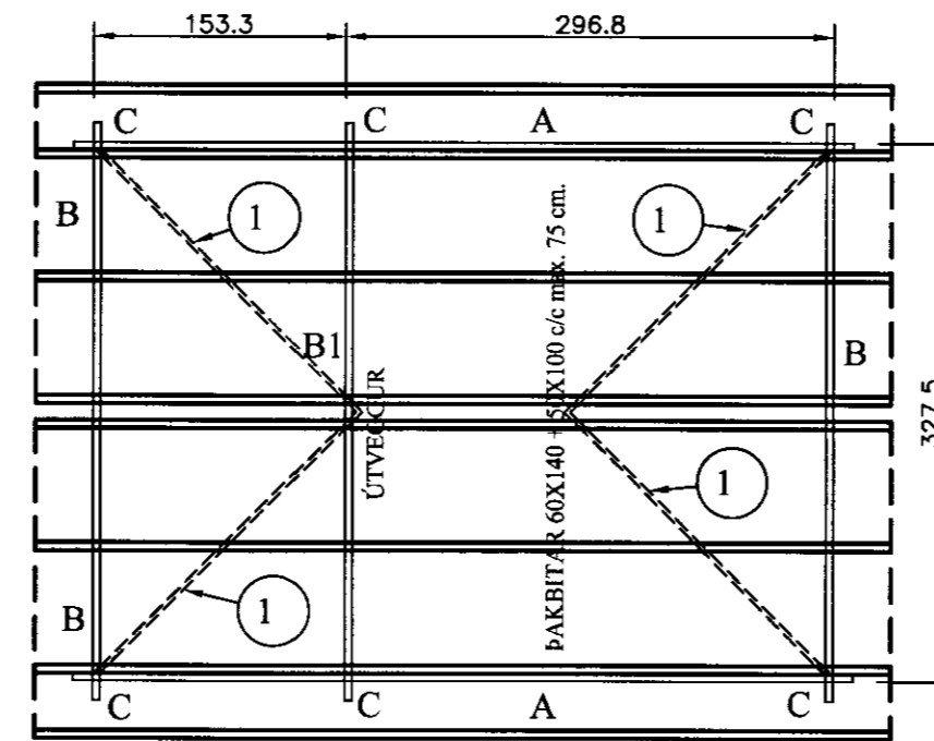
Grunnmynd þak
