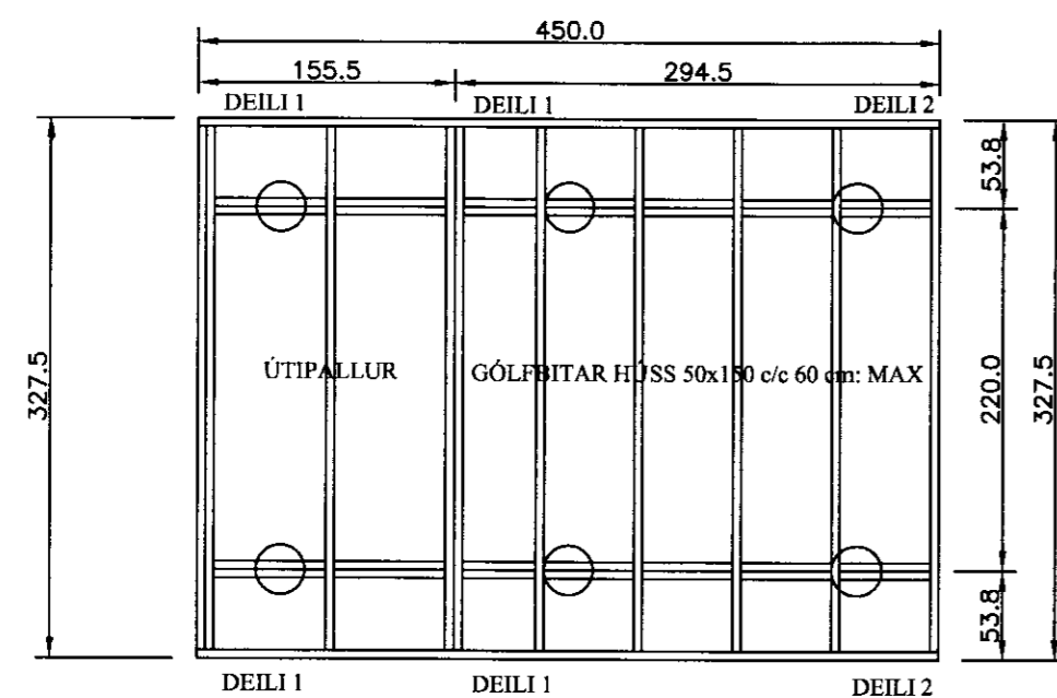
Grunnmynd gólfbitar
