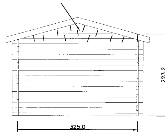
Hliðarmynd gabl festing skásagaðra bjálka
