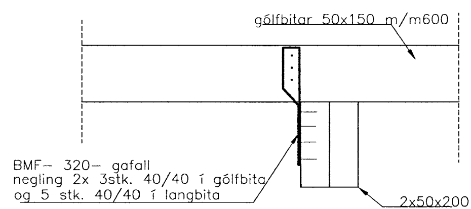
SNIÐ B2 - 1:10
