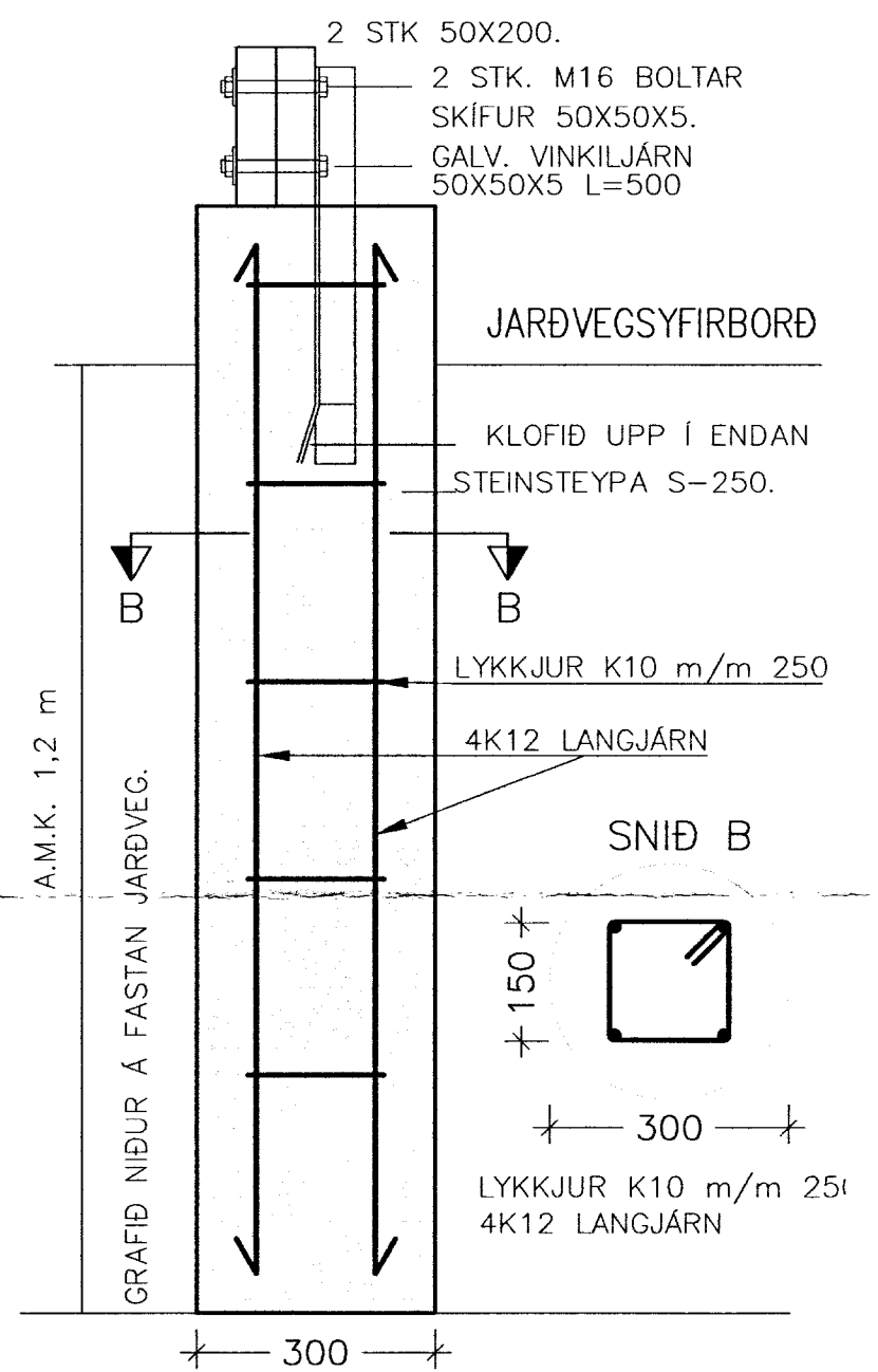
U1- UNDIRSTÖÐUR 1:10
