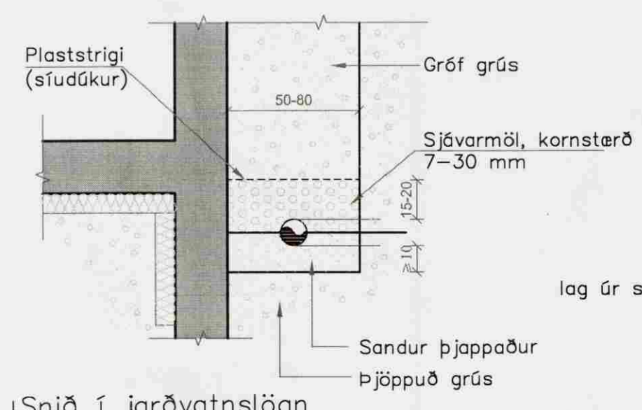
Snið í jarðvatnslögn 1:20
