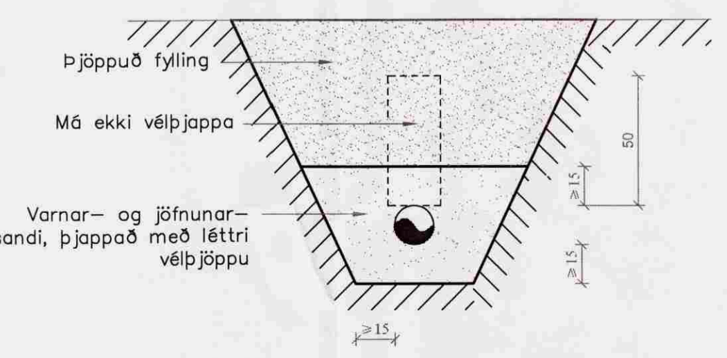
Frárennslislagirnir í jörðu og grunni 1:20
