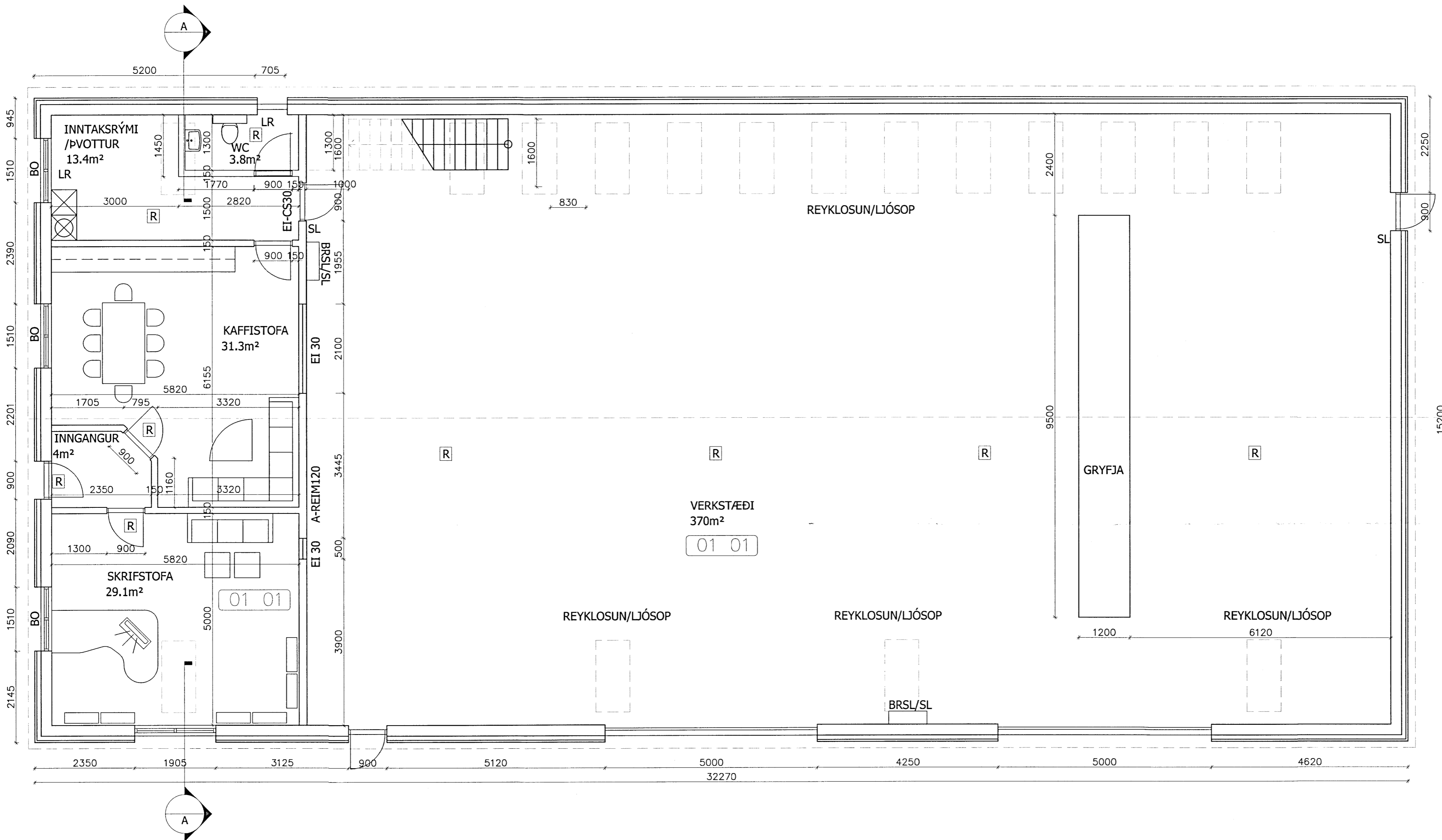
GRUNNMYND JÄRDHÆÐAR 1:50
