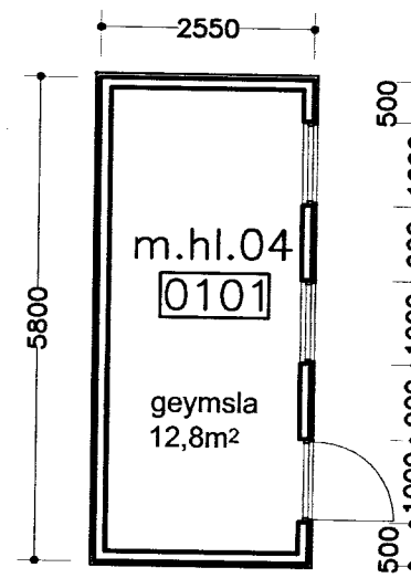
grunnmynd
