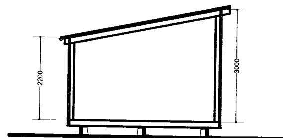
þversnið
