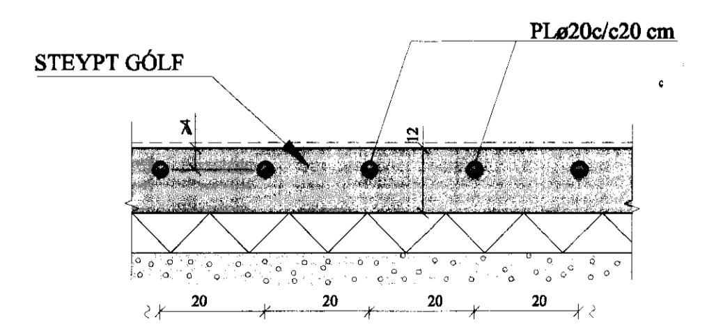
SNIÐ X - X. 1:10
