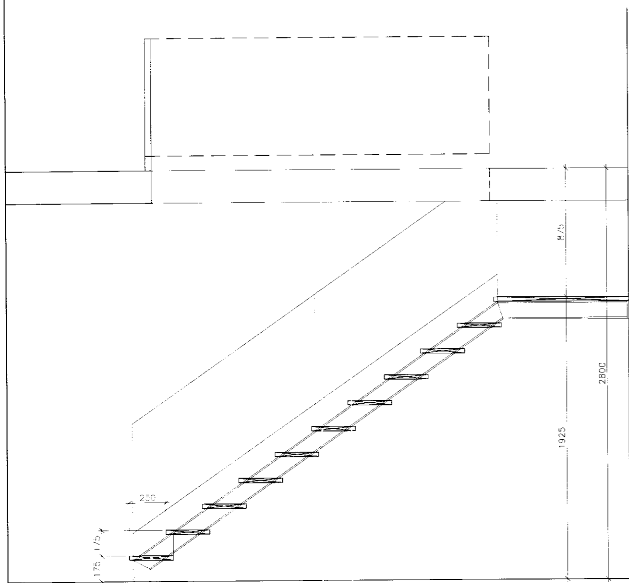
SNID A-A
