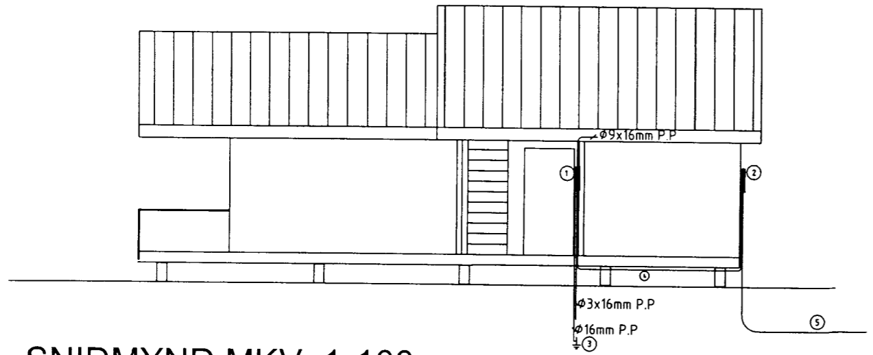
SNIÐMYND MKV. 1-100
