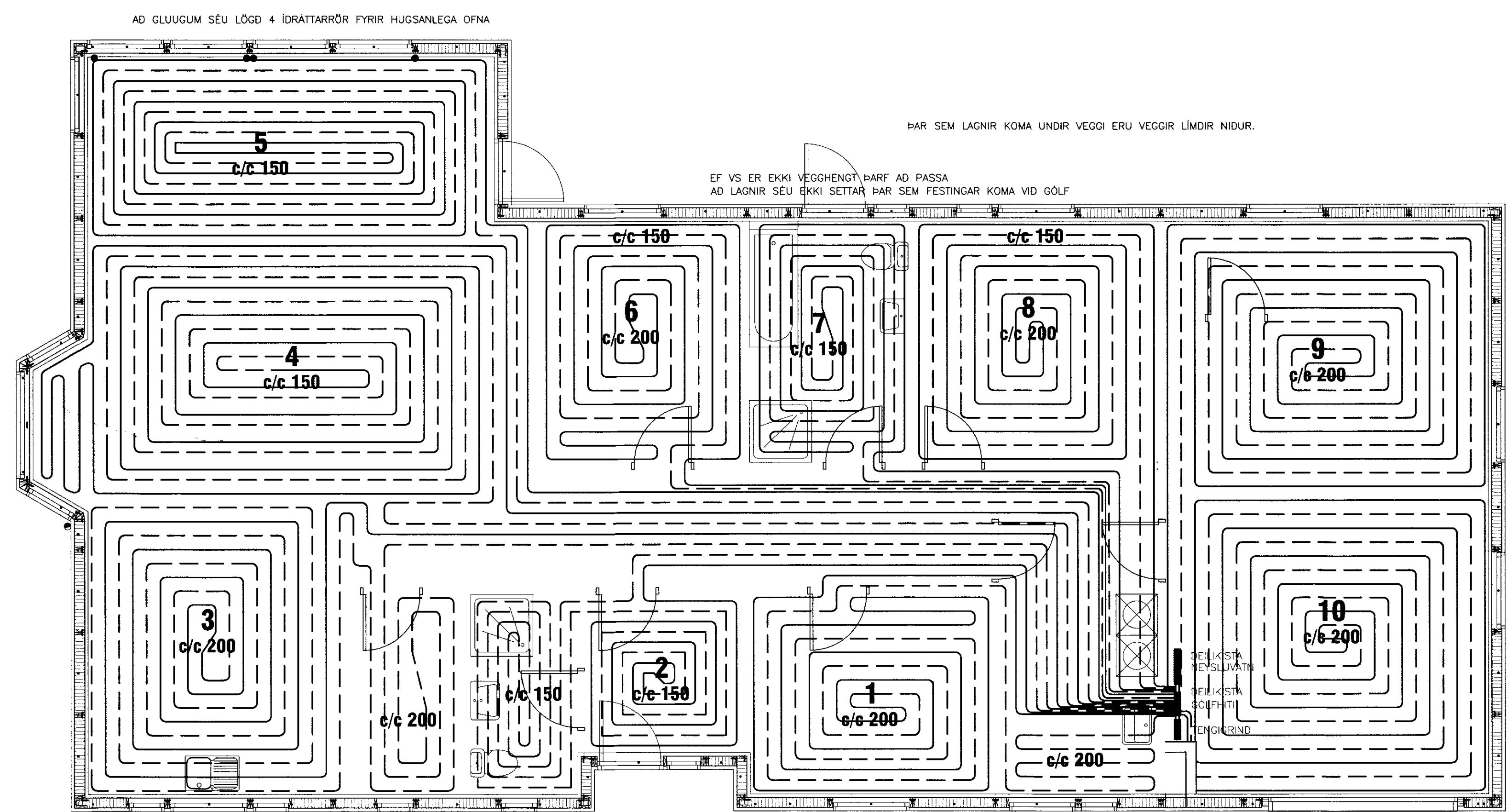
GRUNNMYND GÖLFHITALAGNA MKV. 1:50
