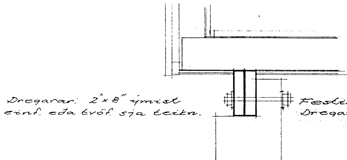
Undirstöður 1:50 (Sjá málsetningu á teikn 102)
