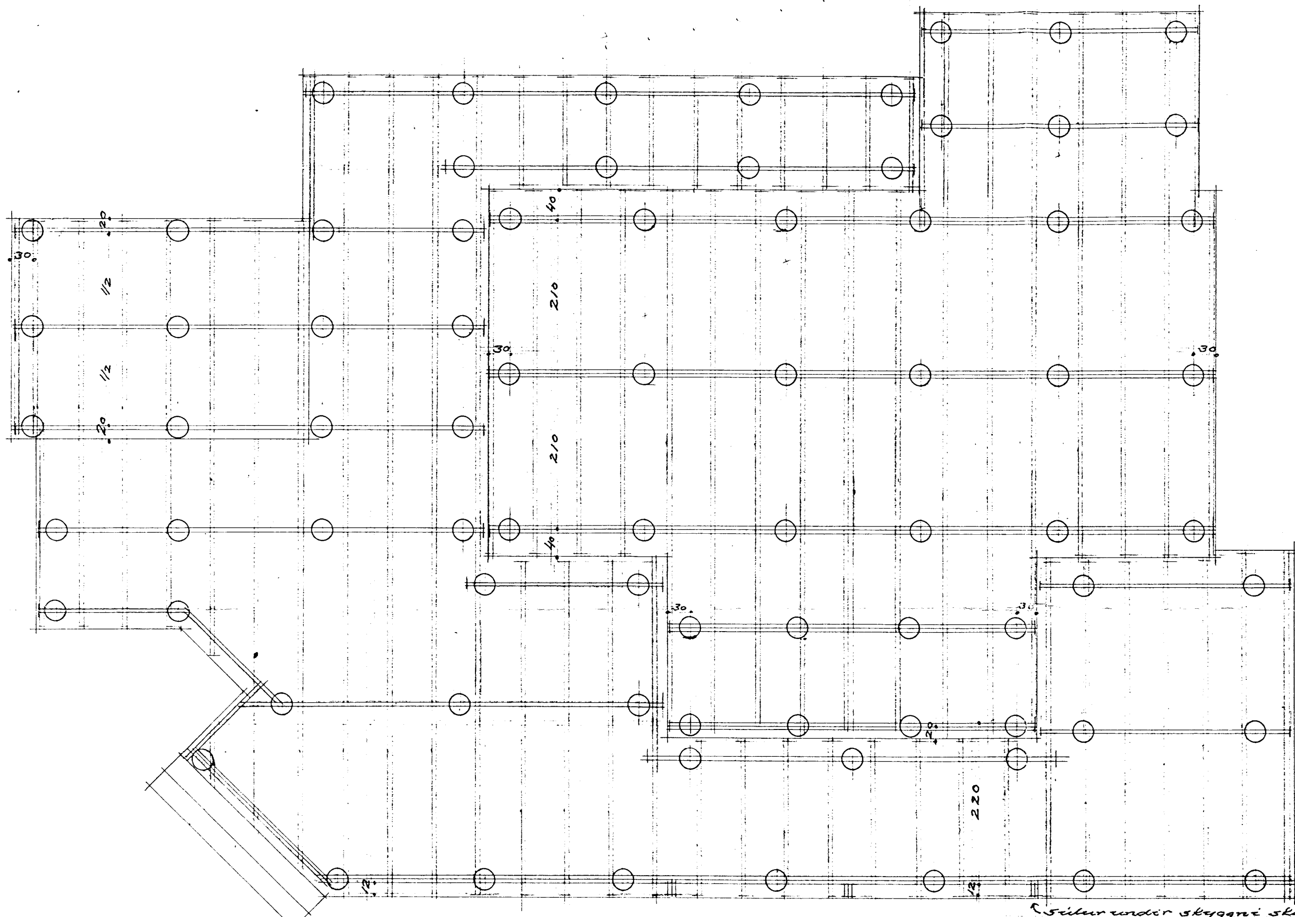
Undirstöður 1:50 (Sjá málsetningu á teikn 102)
