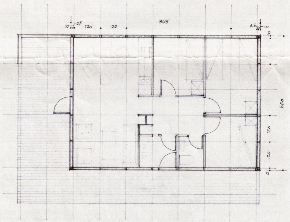
GRUNNMÝND - 1:100
