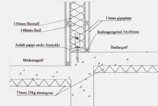
Lóðrétt snið í millivegg (fótstykki) milli íbúðar og bilageymslu
