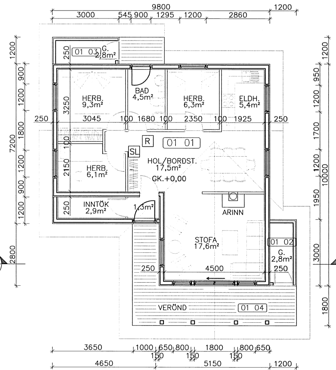
GRUNNMYND 1:100
